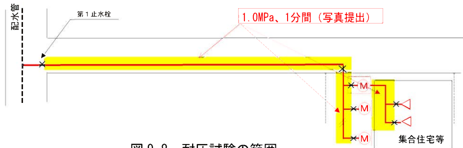
図 9-8 耐圧試験の範囲
