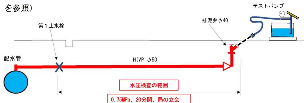
図 9-9 \phi 40 以上の耐圧試験 ( \phi 50 の場合の例)
