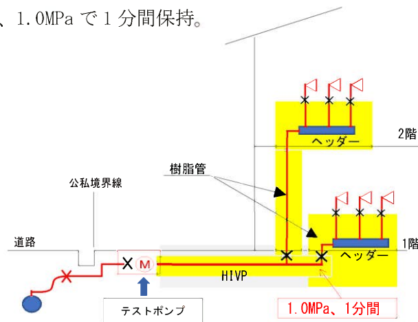
図 9-7 耐圧試験の範囲
