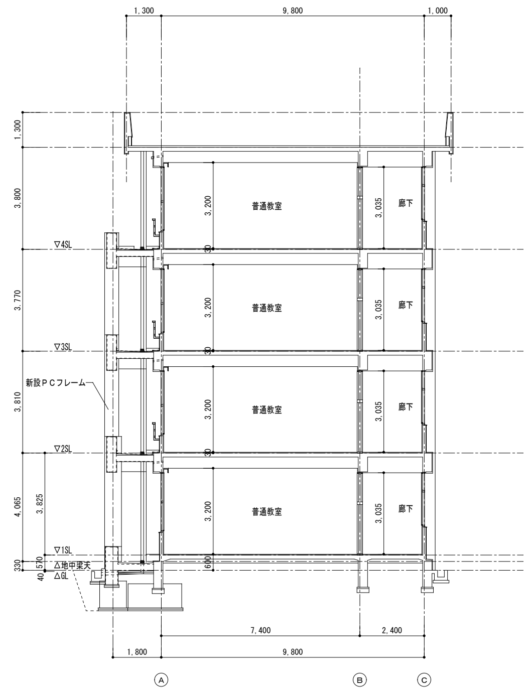
改修後断面図 1/100
