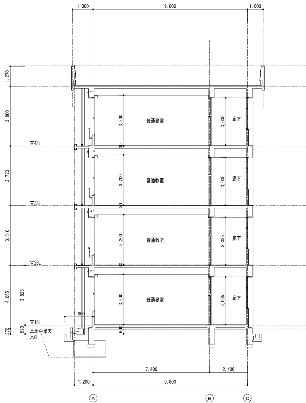
現況断面図 1/100
