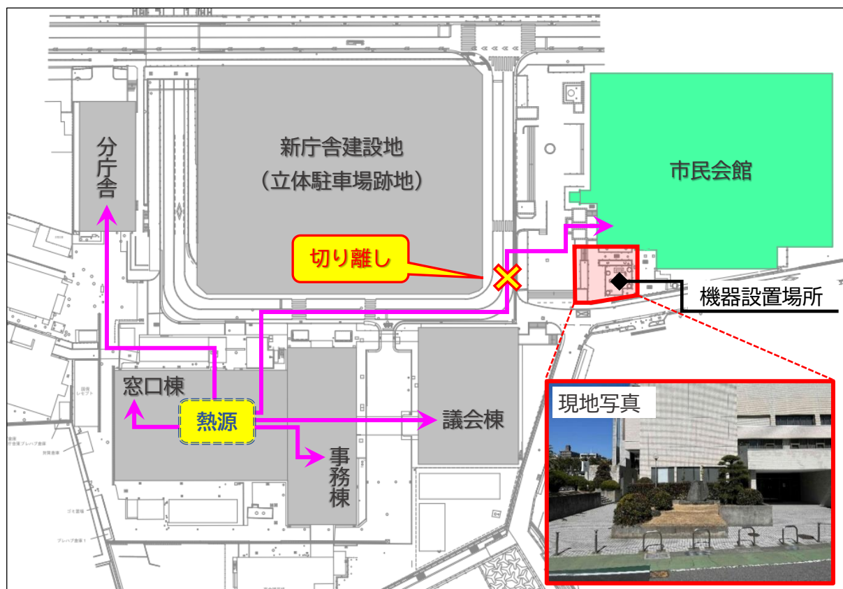
空調系統平面図
