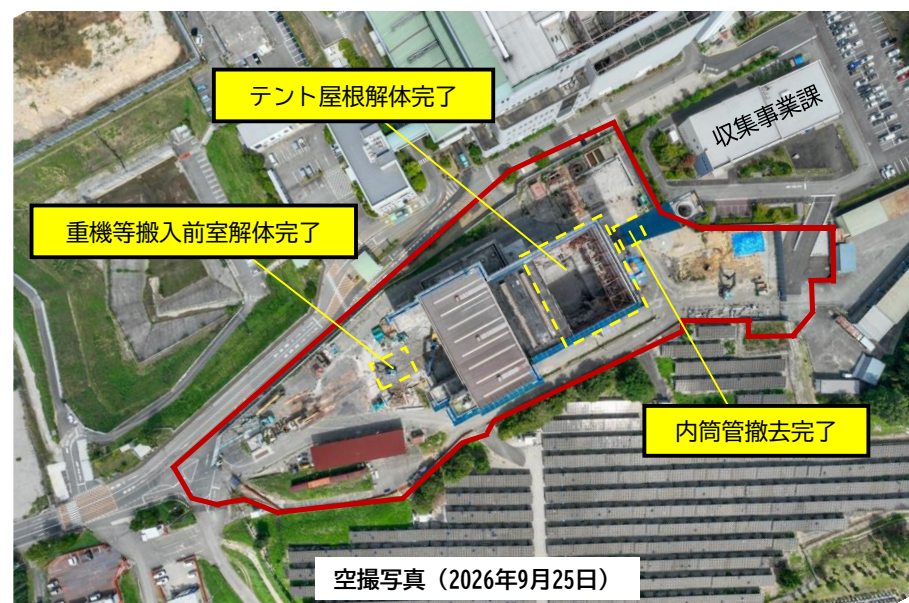
⑤ テント屋根 解体状況
