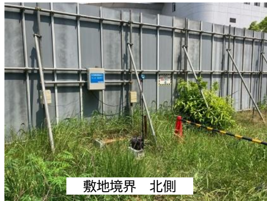
④ 煙突耐火材撤去に伴う 環境調査状況
