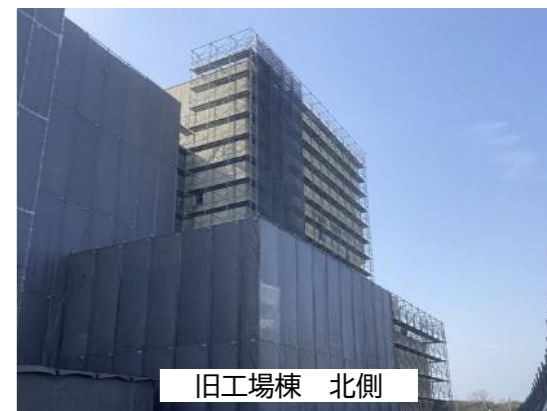
④外部養生足場設置状況
