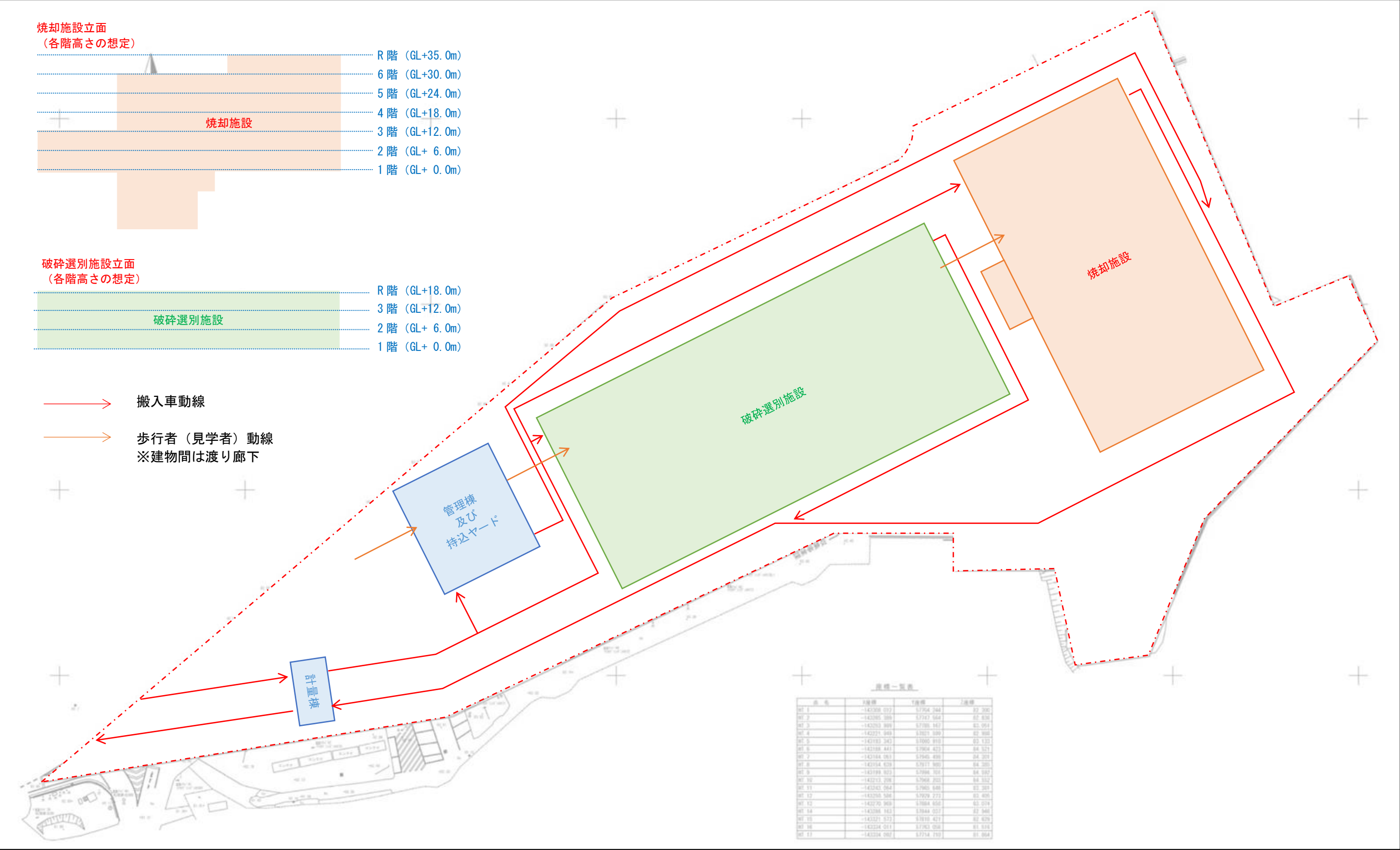
図 6-4 全体施設配置イメージ
