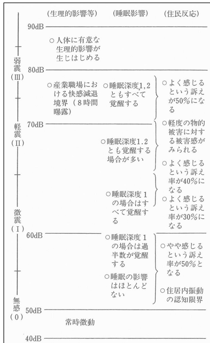
図 5-2 振動の目安
