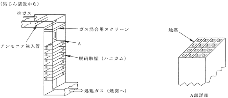
図 触媒脱硝反応塔
