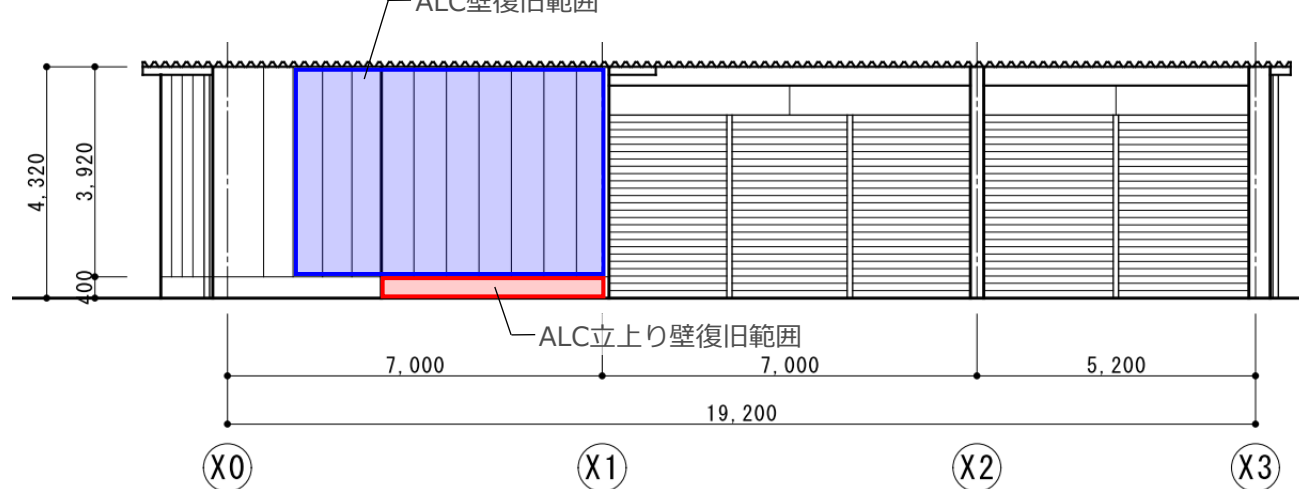
南立面図
