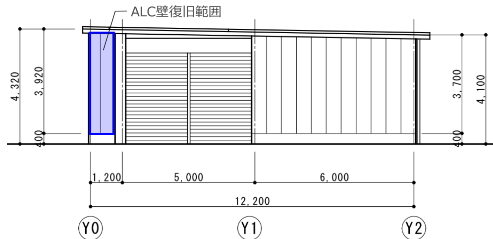
東立面図
