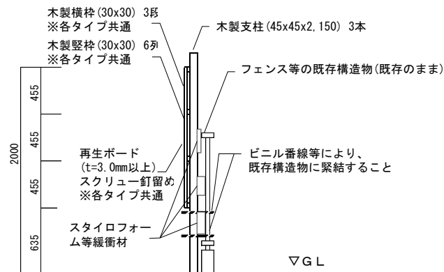
A タイプ断面図 (参考) 1/30
