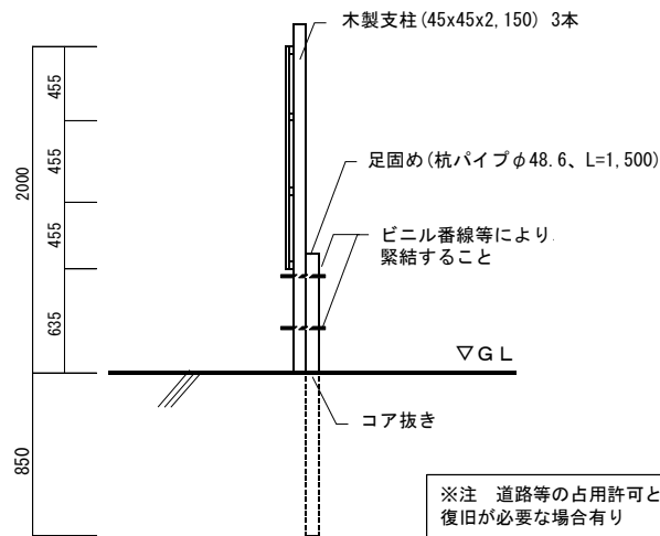
C タイプ断面図 (参考) 1/30
