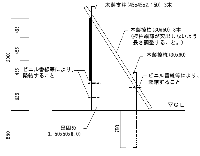
B タイプ断面図 (参考) 1/30
