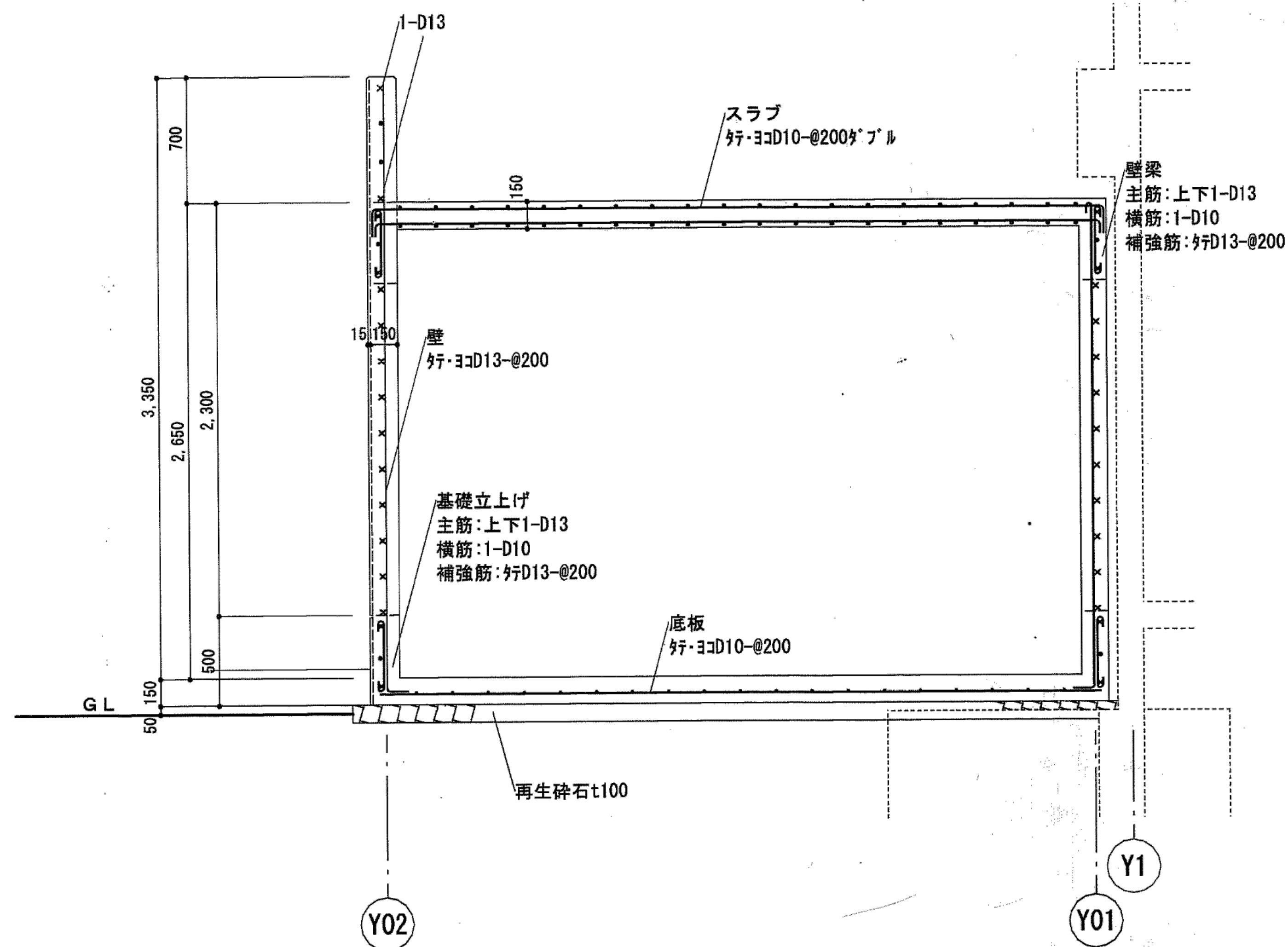
消毒室 配筋図 S=1/30
