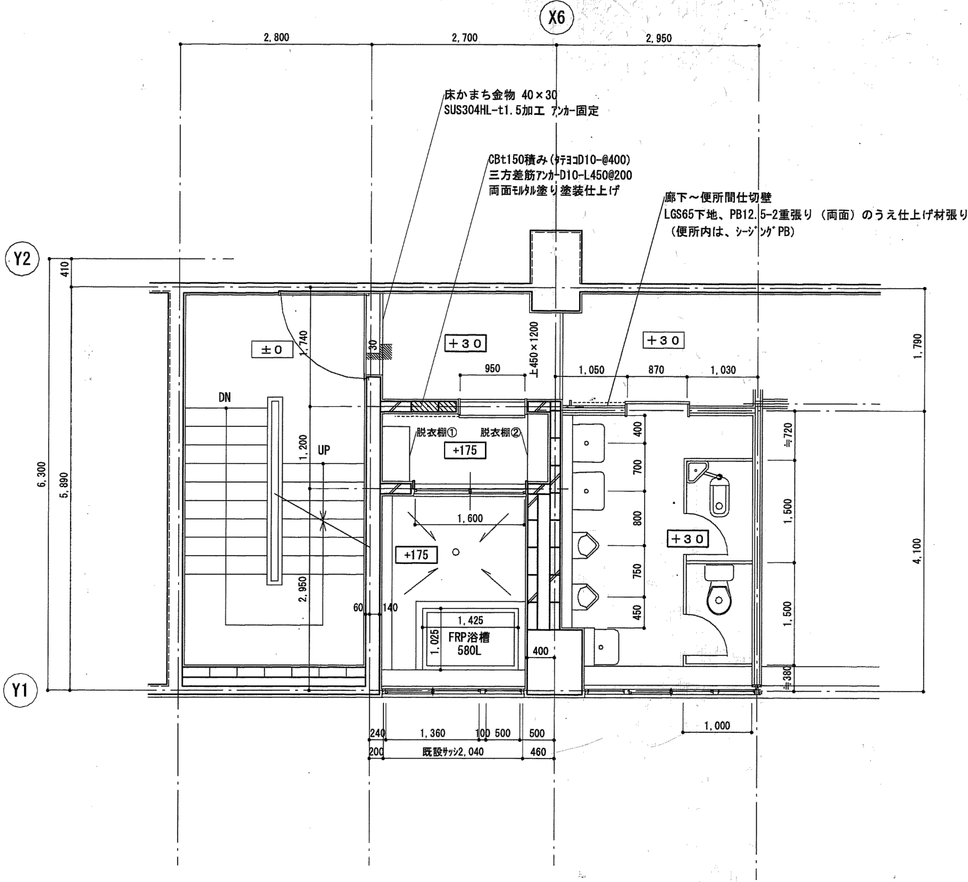
風呂・便所 平面詳細図 S=1/50
