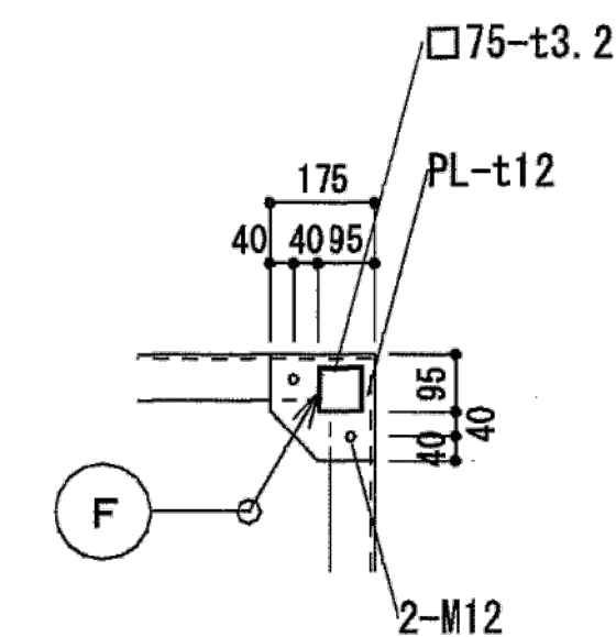
踊り場支柱見上げ図 S=1/20
