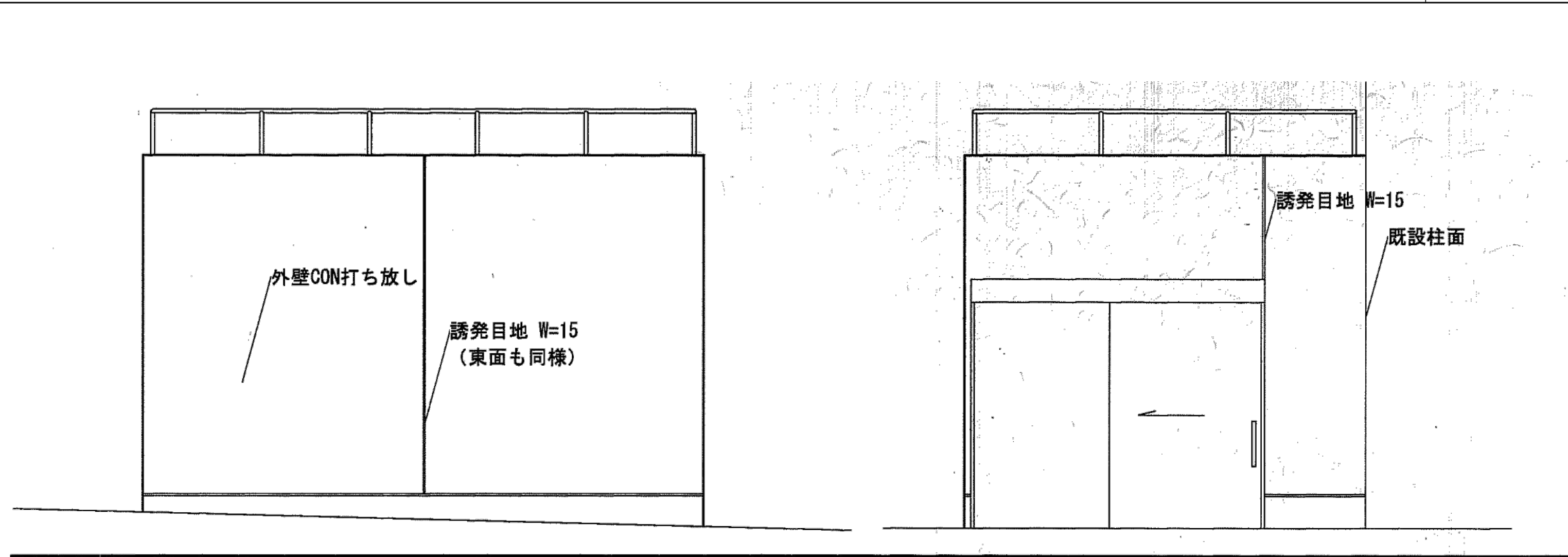
北 立面図 S=1/50
