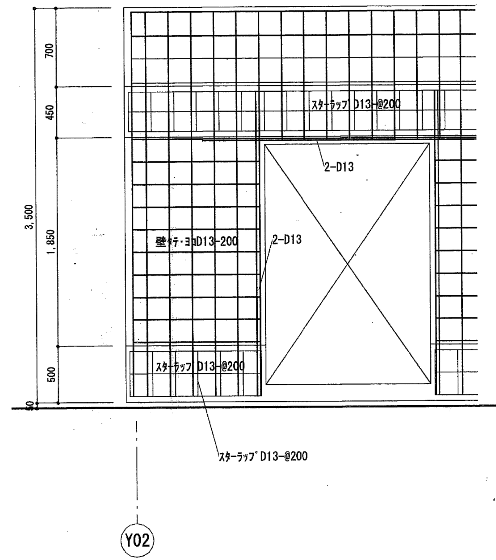
X01通り配筋図 S=1/30
