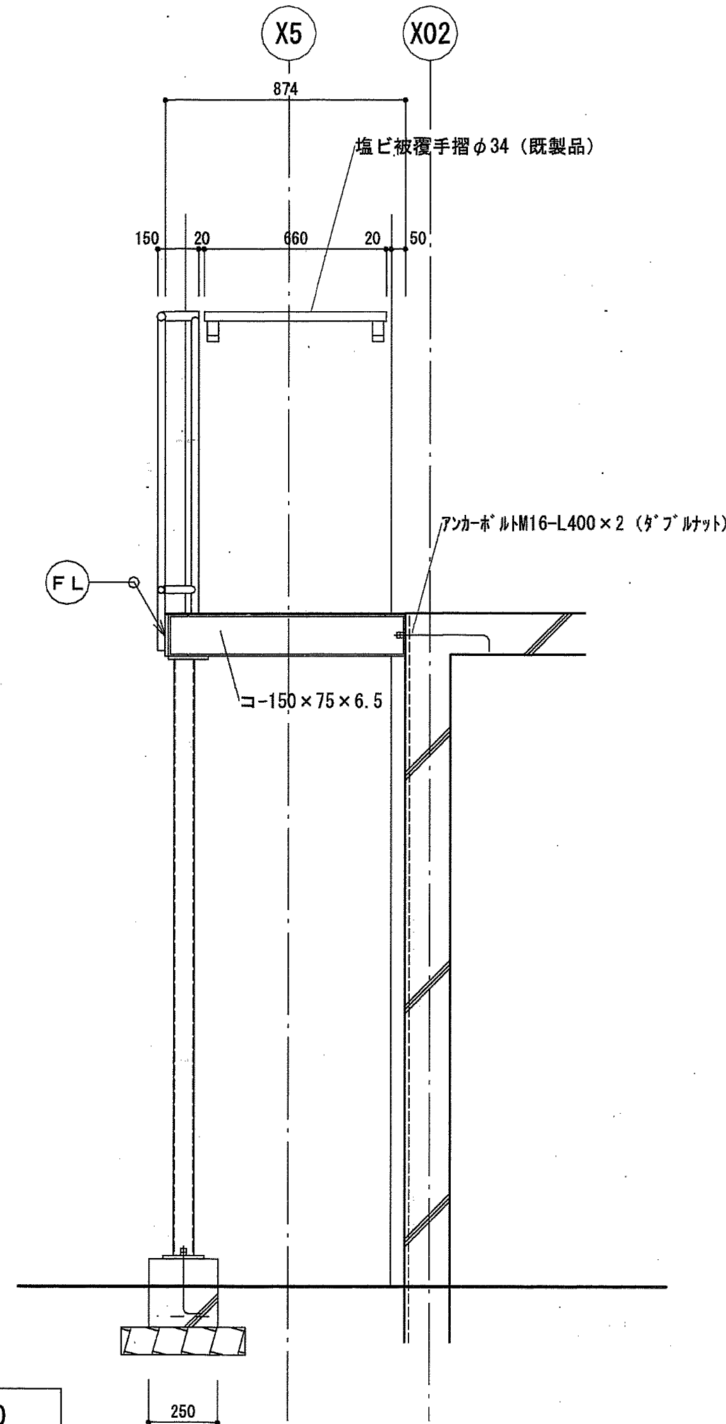
階段断面図 S=1/20
