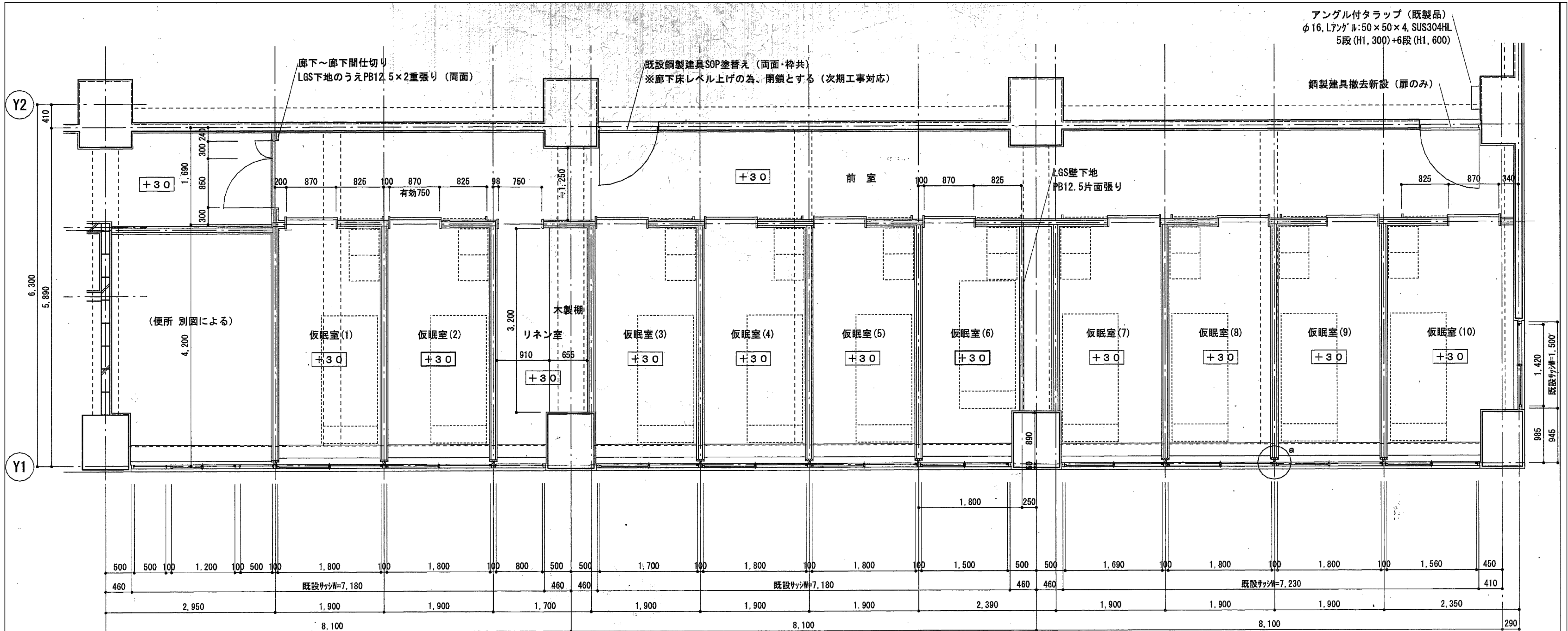
仮眠室廻り平面詳細図 S=1/50
