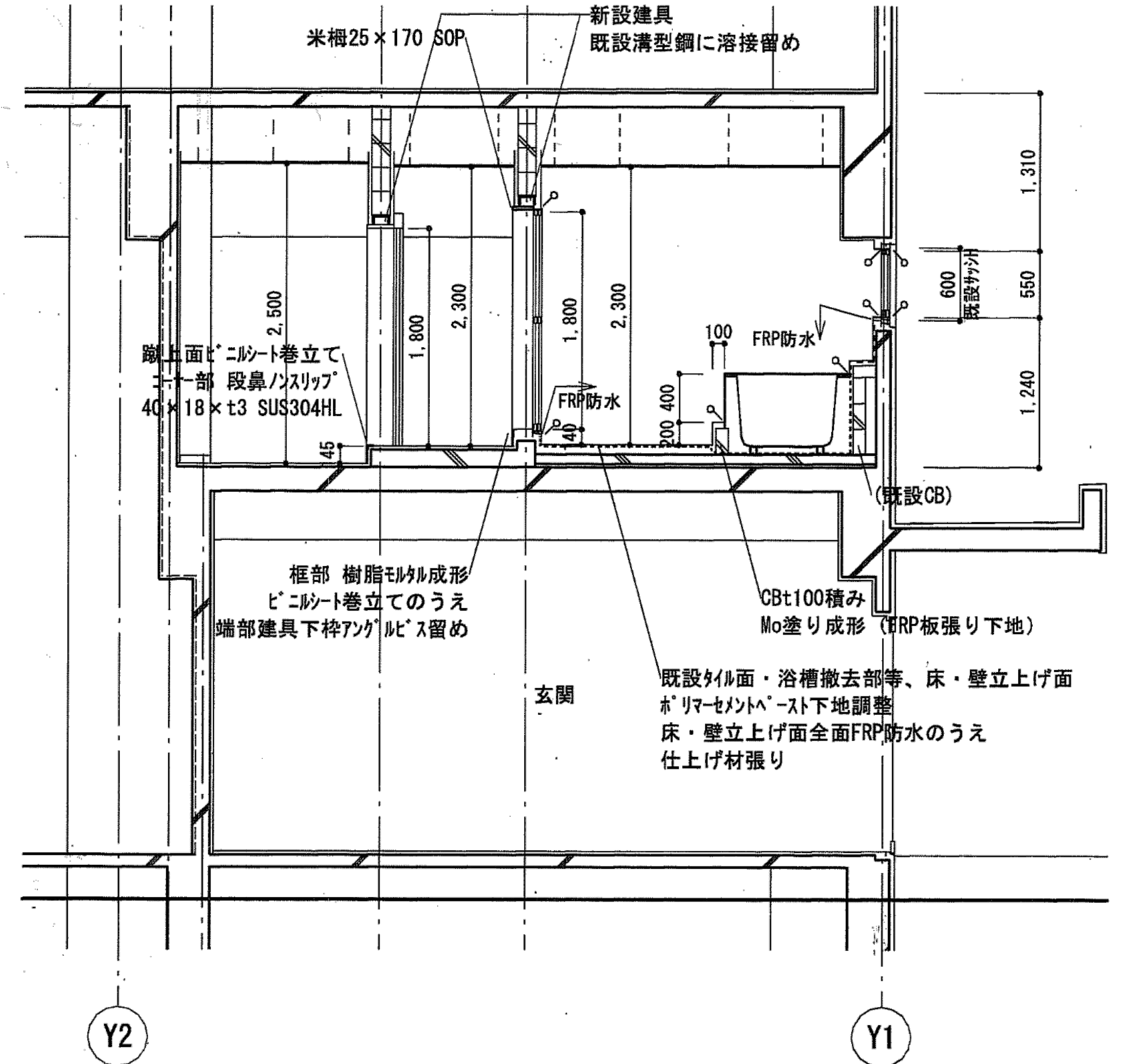
X方向 断面詳細図 S=1/50
