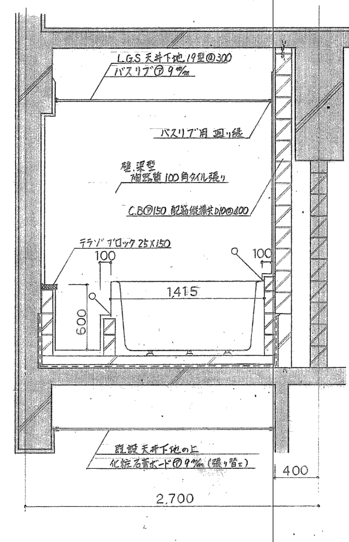
X-X' 断面詳細図 (改修後) S = 1/30
