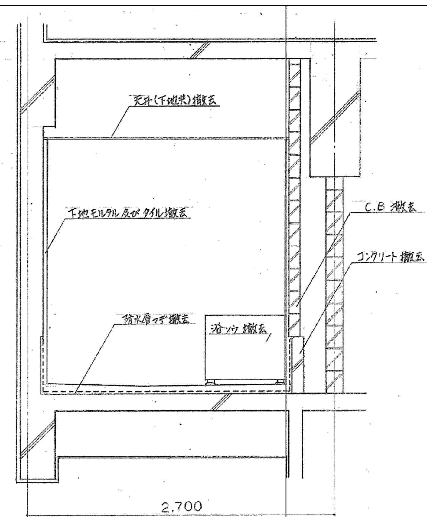
X-X' 断面詳細図 (改修前) S = 1/30
