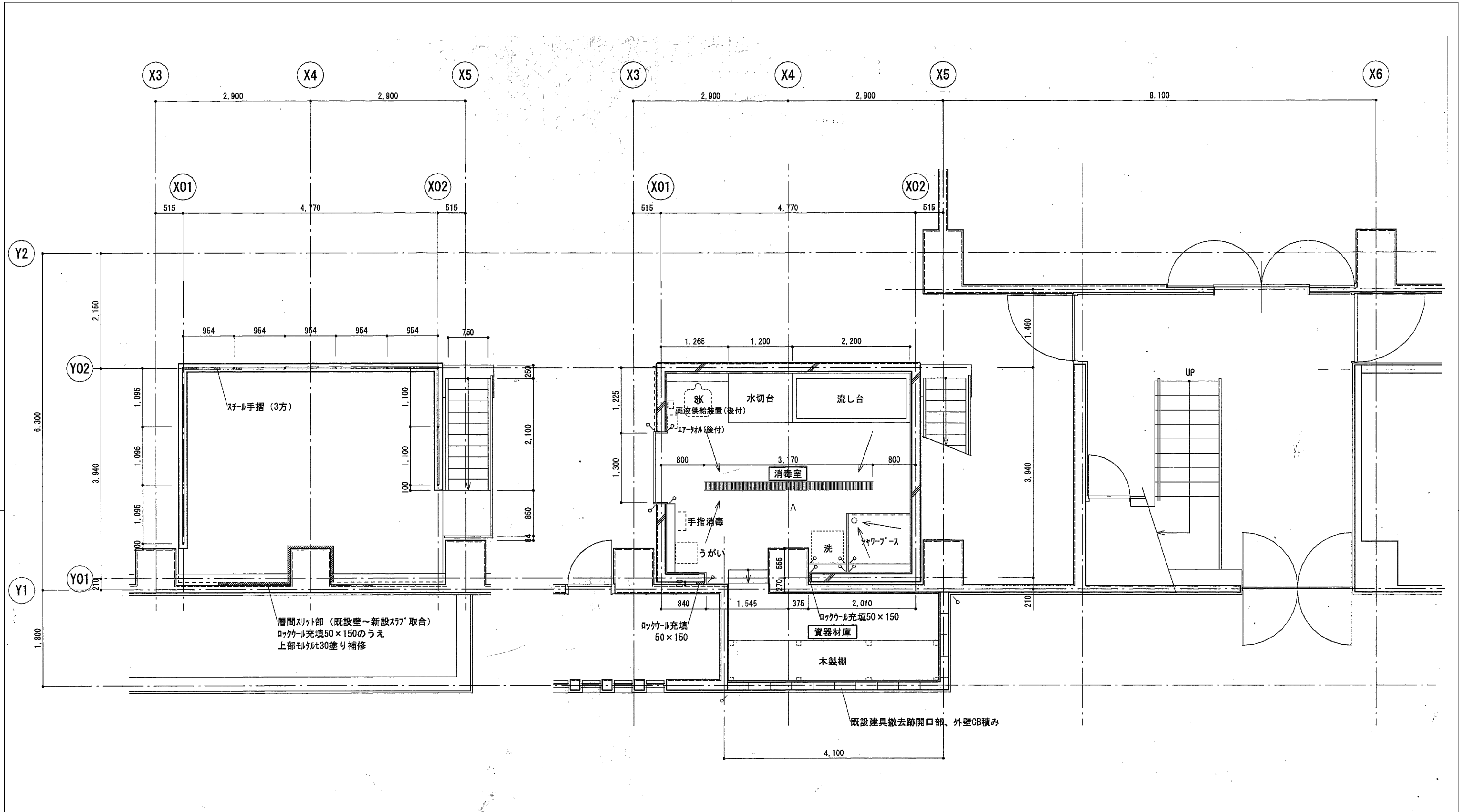
消毒室屋上伏せ図 S=1/50
