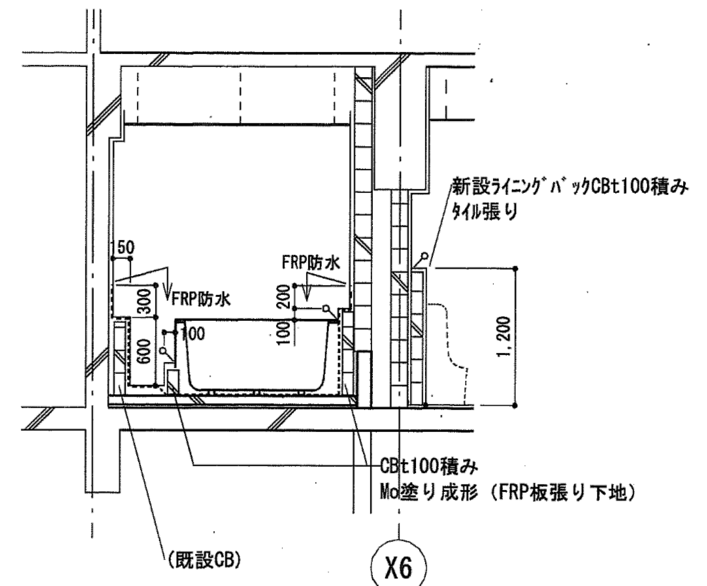
Y方向 断面詳細図 S=1/50
