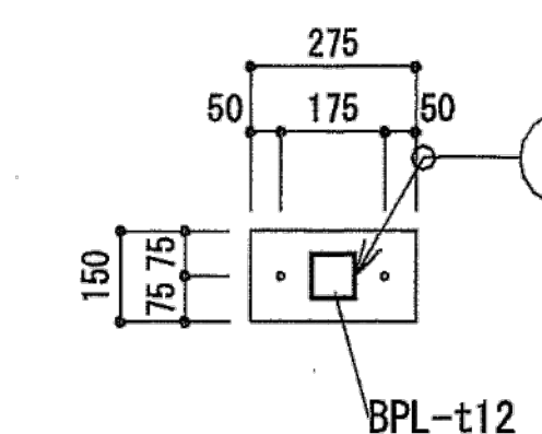
ベースプレート S=1/20
