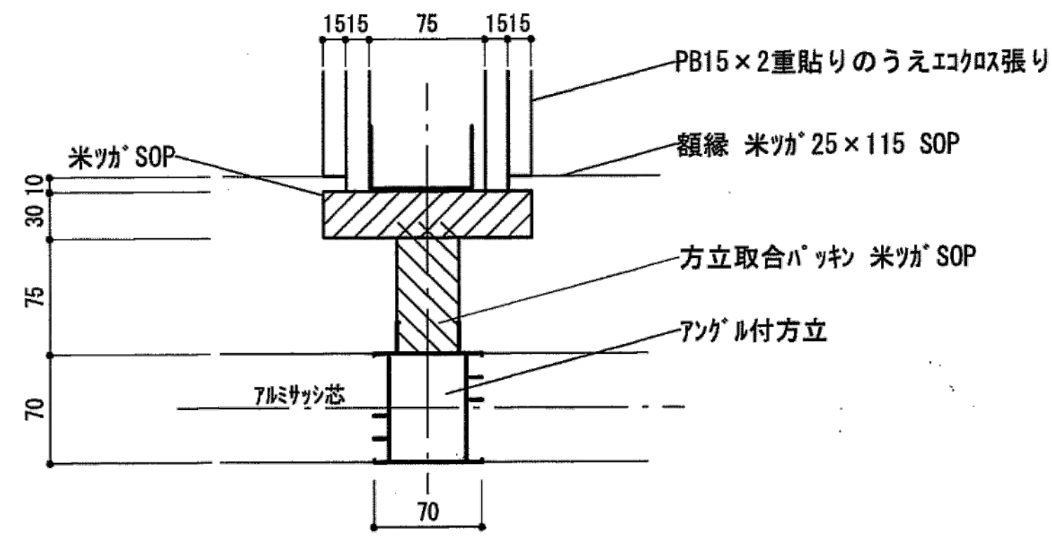
a部詳細図 S=1/5
