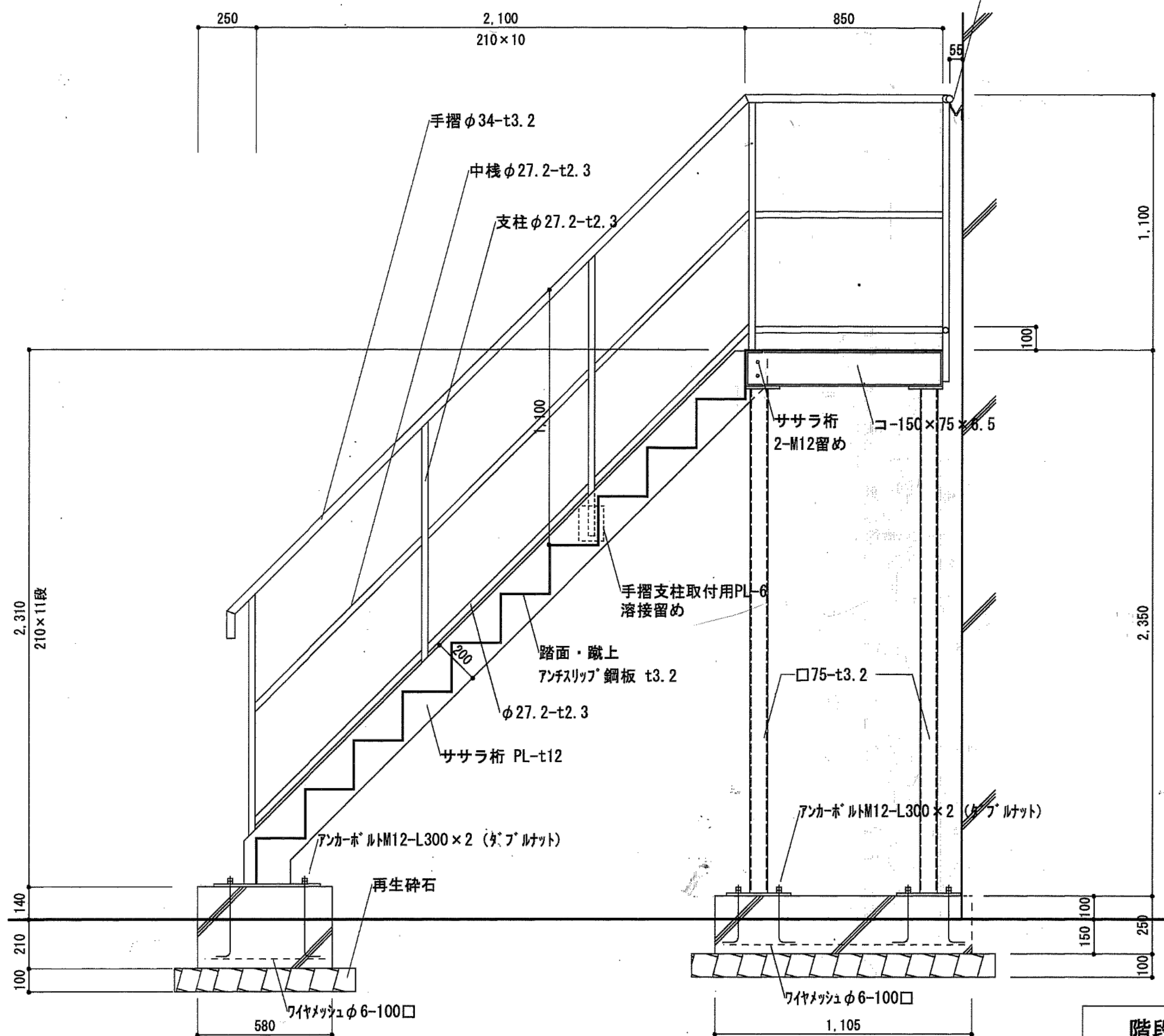
階段平面図 S=1/20
