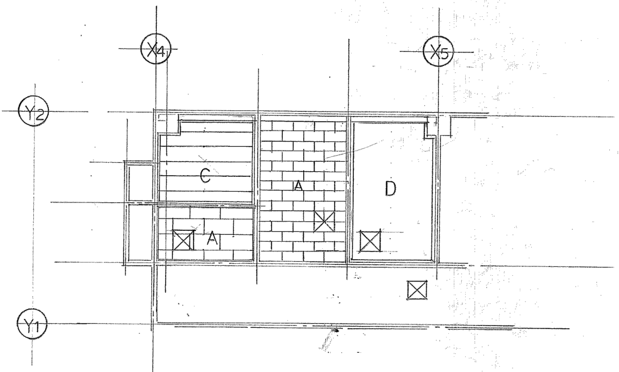
2階天井伏図 1/100
