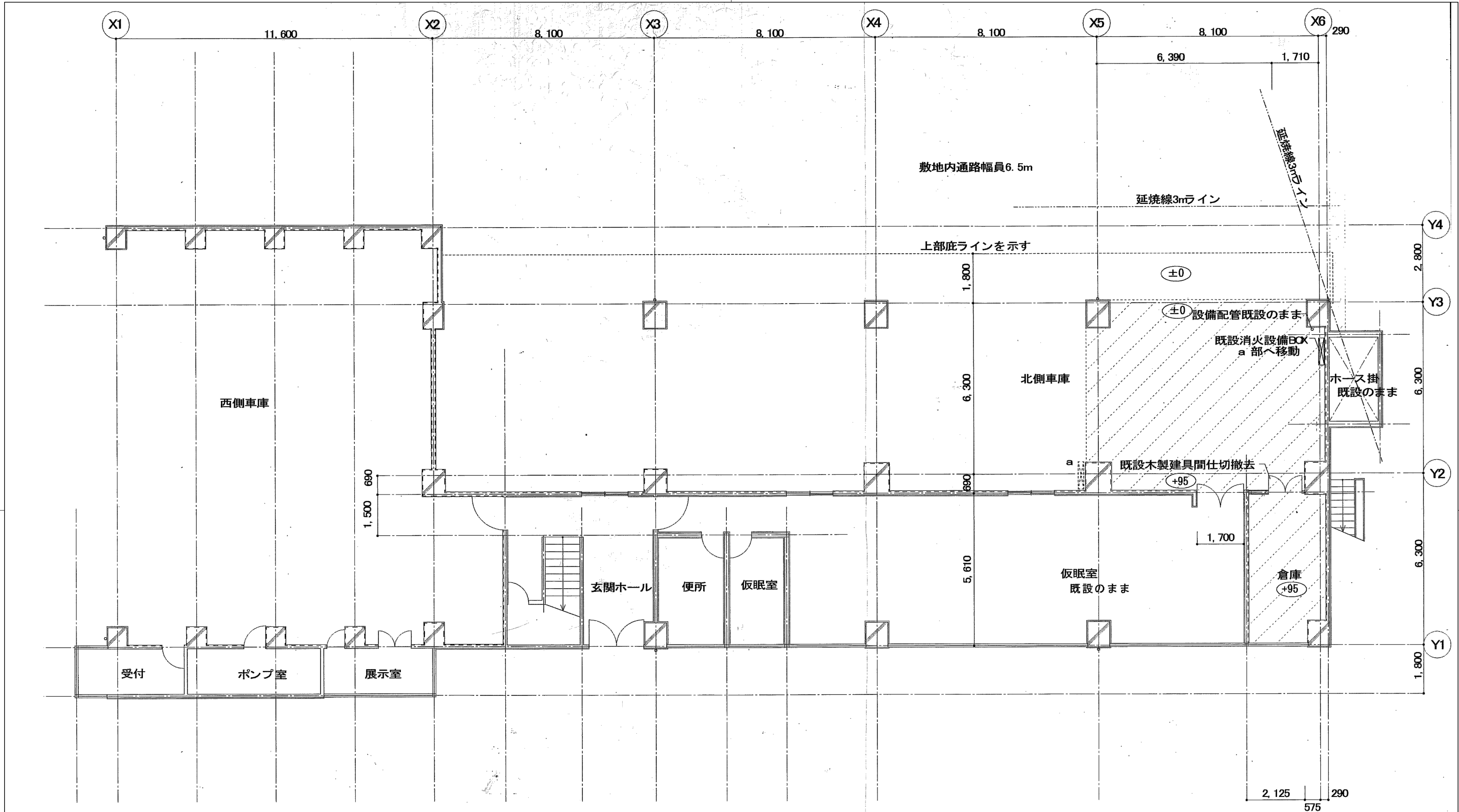
既設1階平面図 1/100
