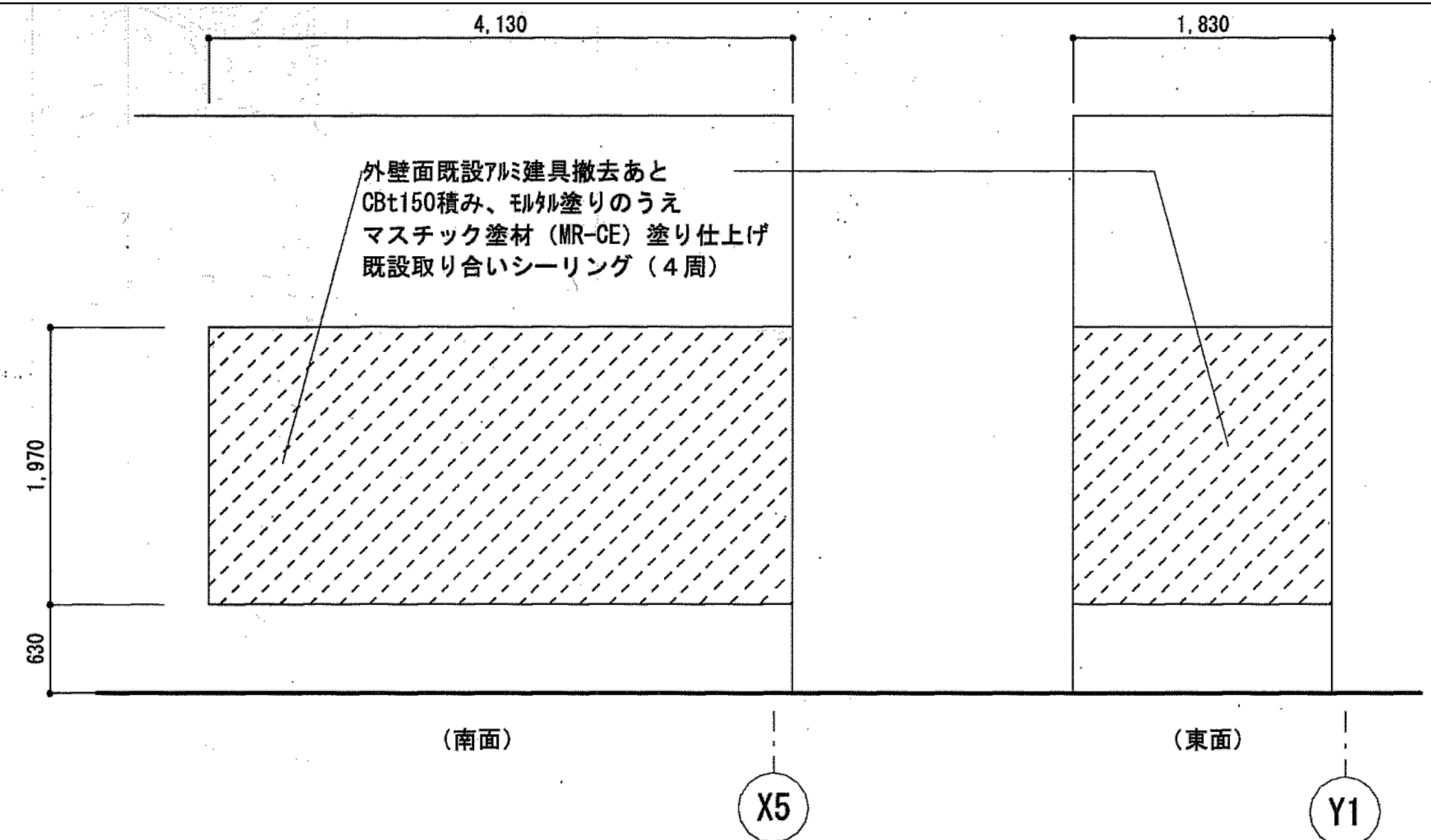
資器材庫外壁立面図 S=1/50
