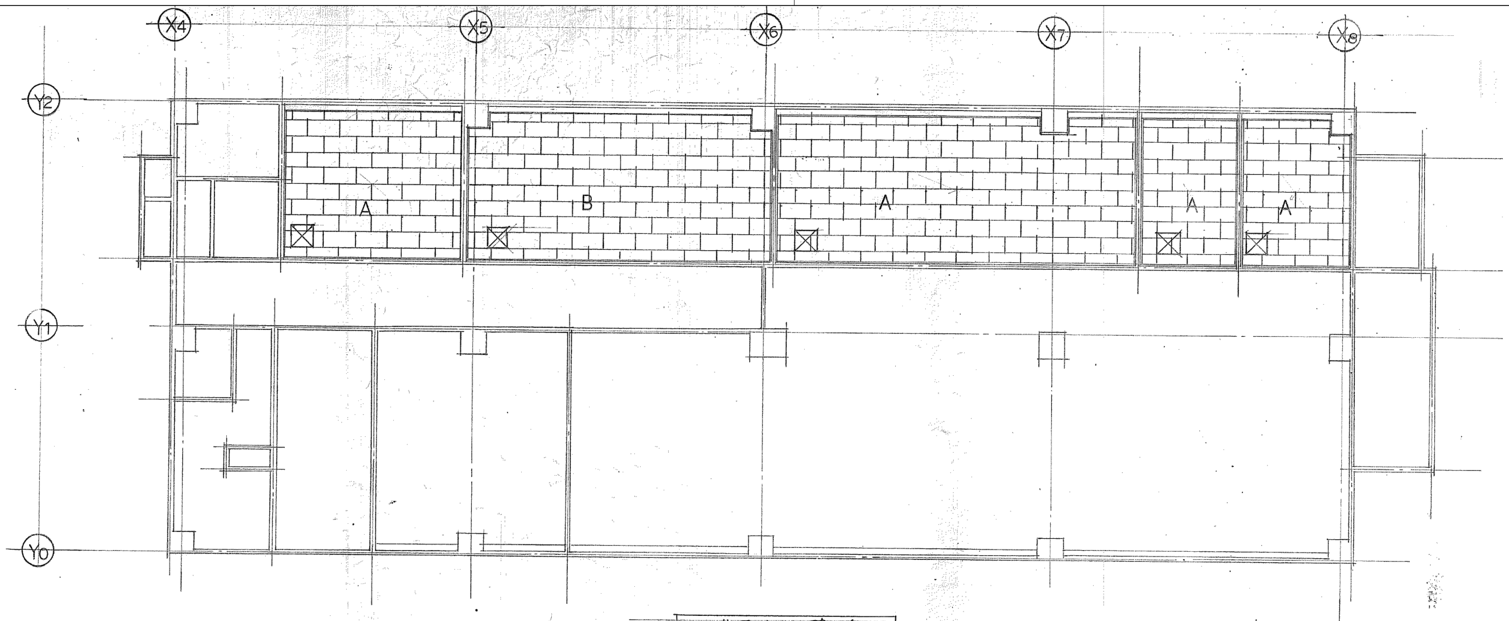
3階天井伏図 1/100
