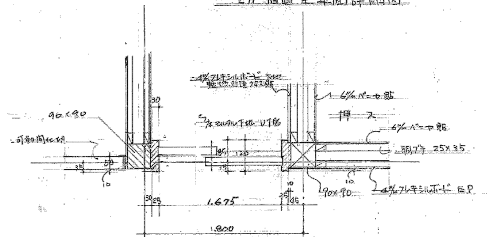
2H 宿直室平面詳細図
