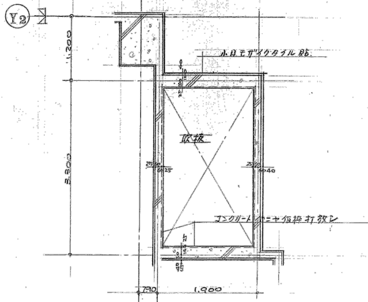
2階平面詳細 1/50
