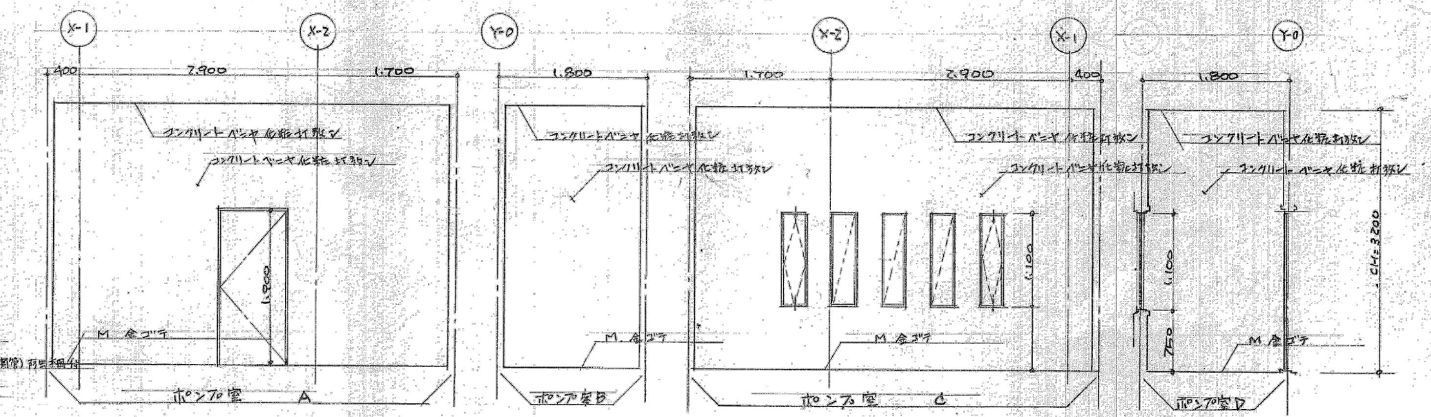
ポンプ室 断面 1/50
