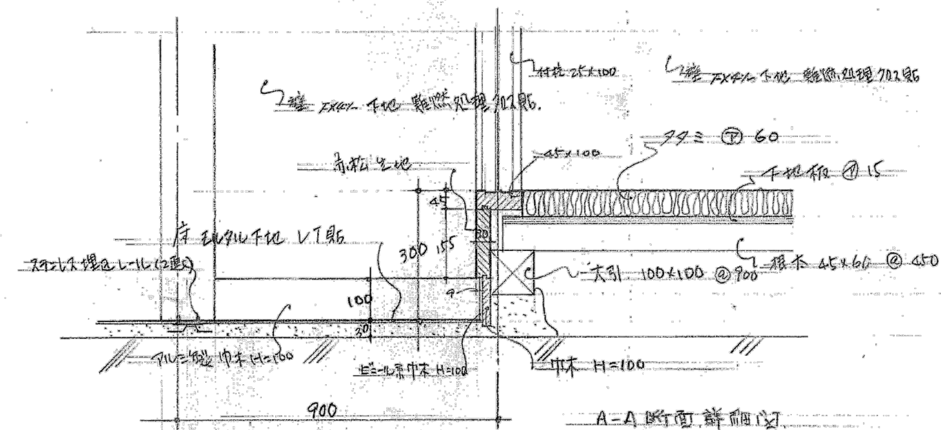
A-A 断面詳細図
