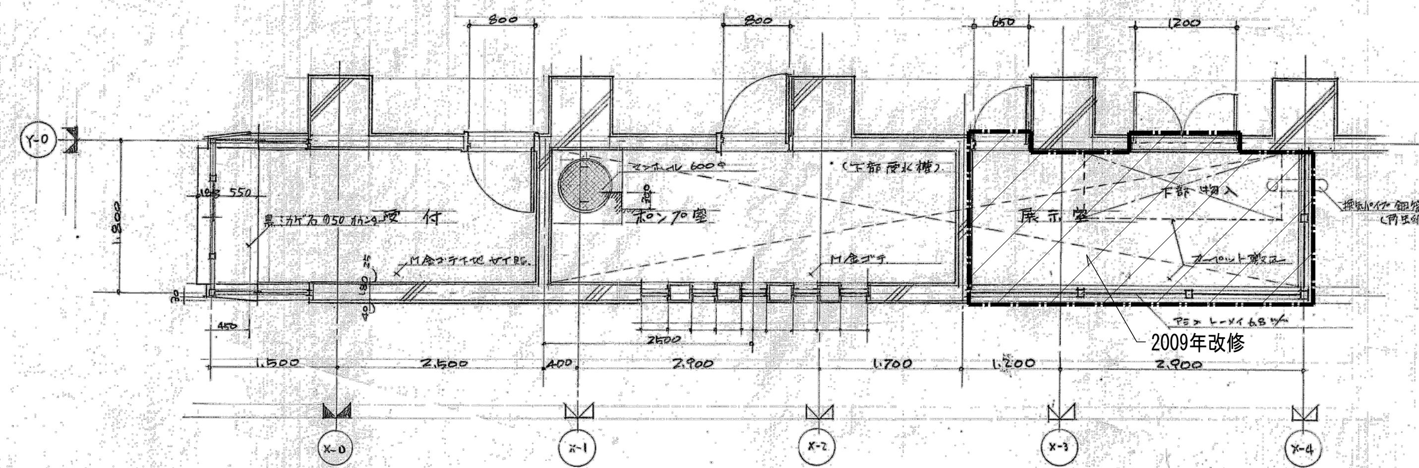
受付・ポンプ室・展示室平面詳細 1/50
