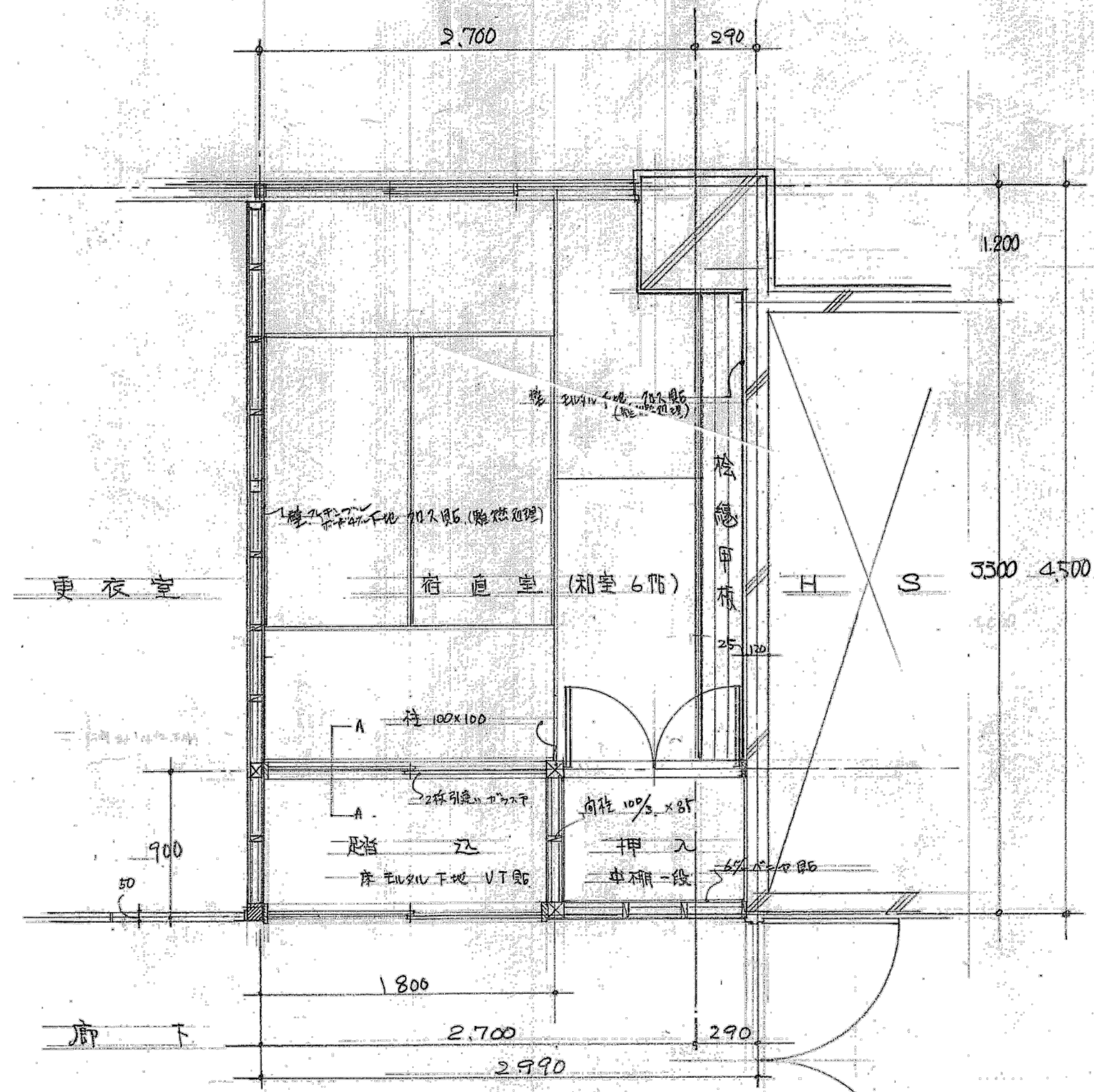
2H 宿直室平面詳細図
