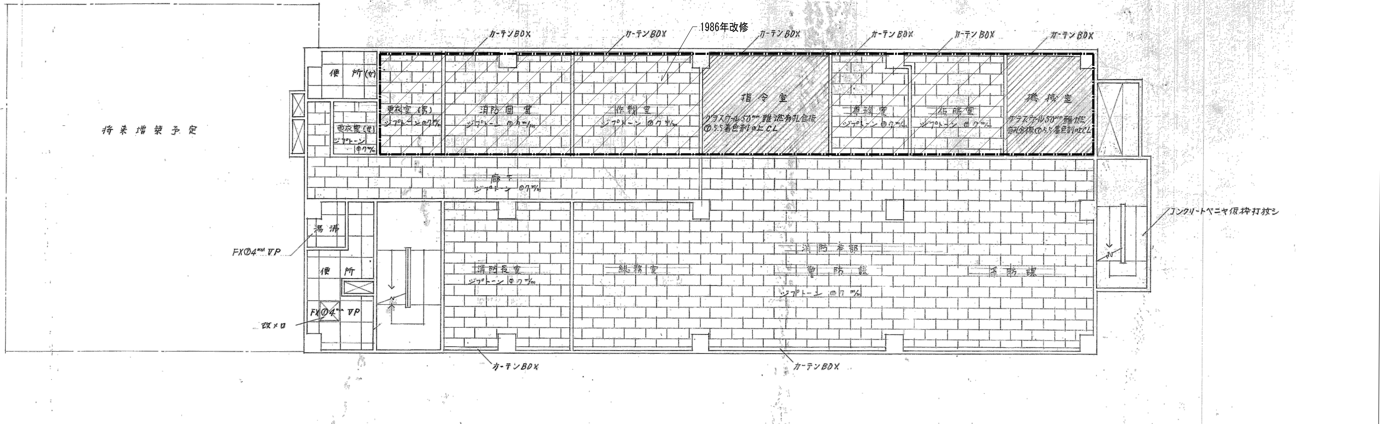
3階 天井伏図
