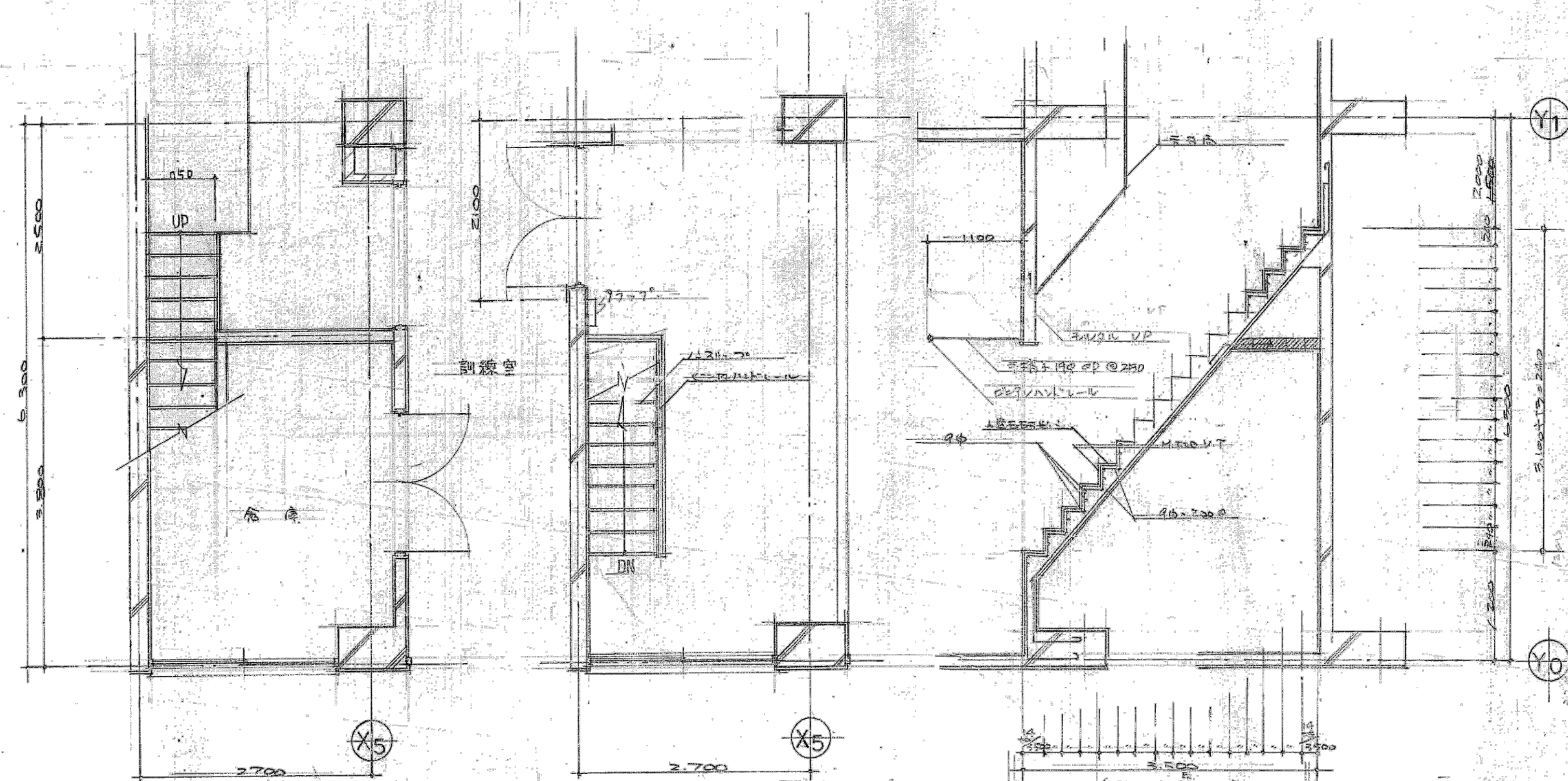
4階階段詳細図
