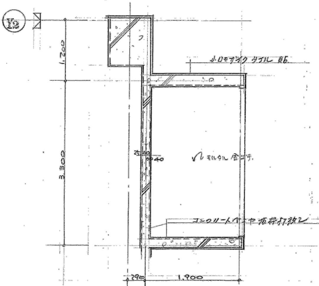
3階平面詳細 1/50
