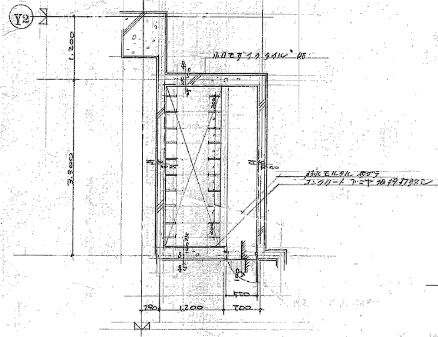
1階平面詳細 1/50
