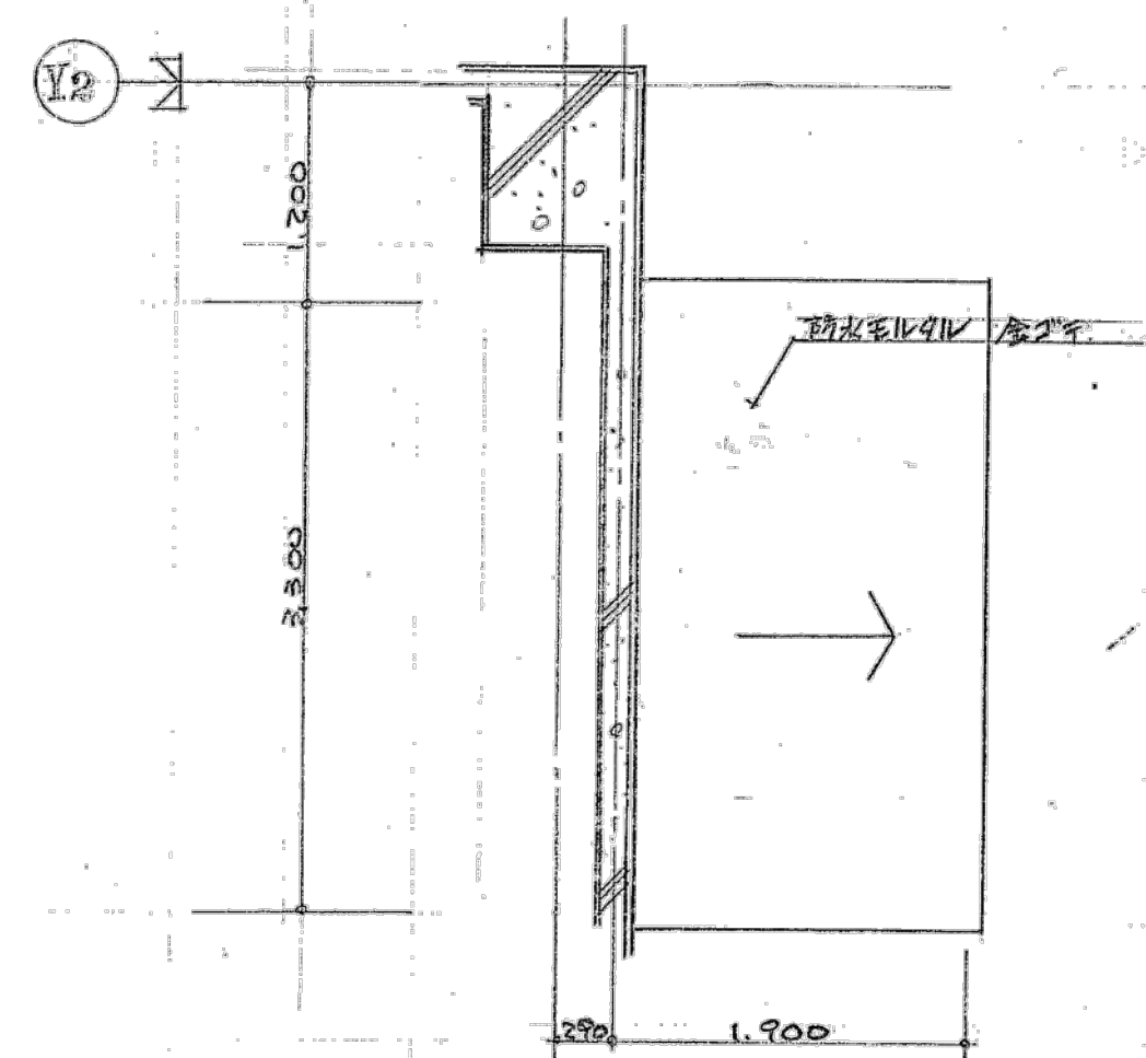
屋根平面詳細 1/50
