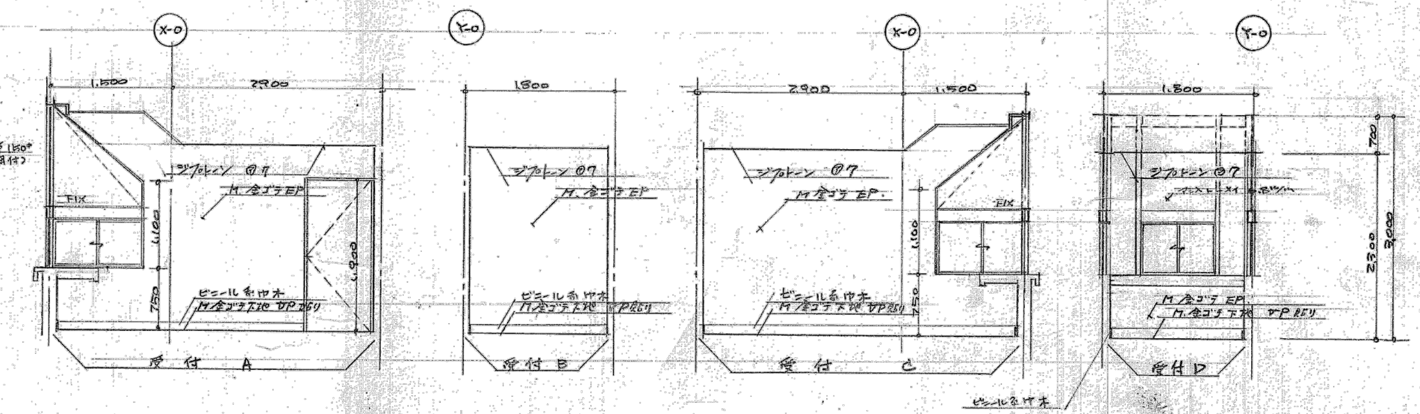
受付・展示室 1/50
