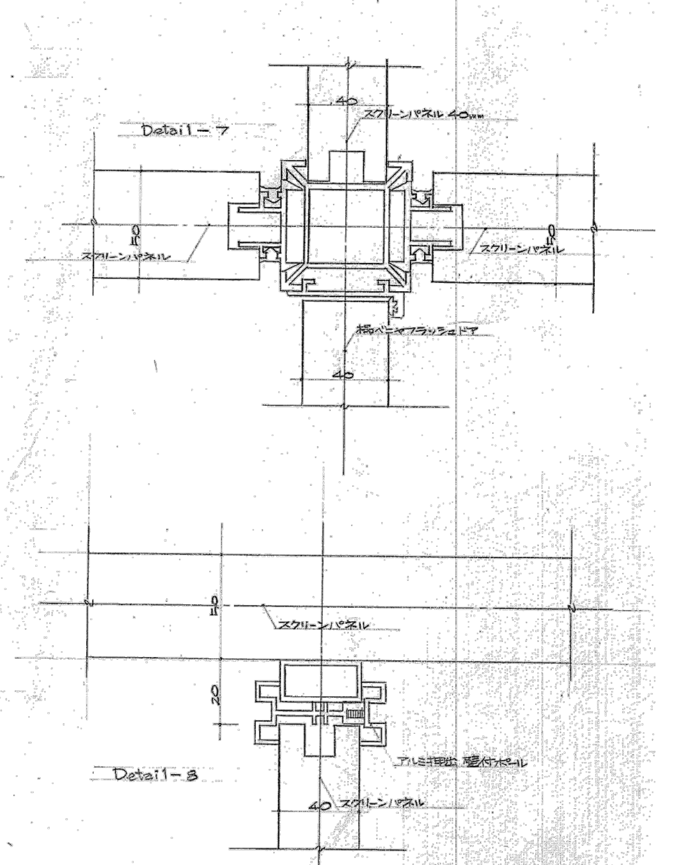
スクリーンパネル詳細図 S:1/2
