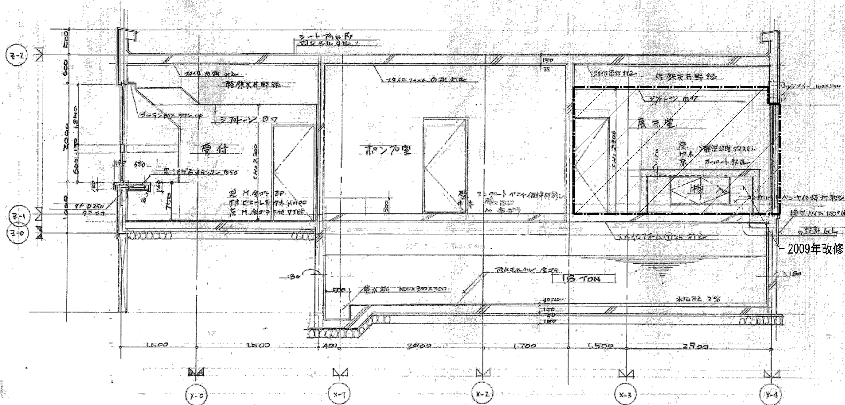
受付・ポンプ室・展示室断面詳細 1/50
