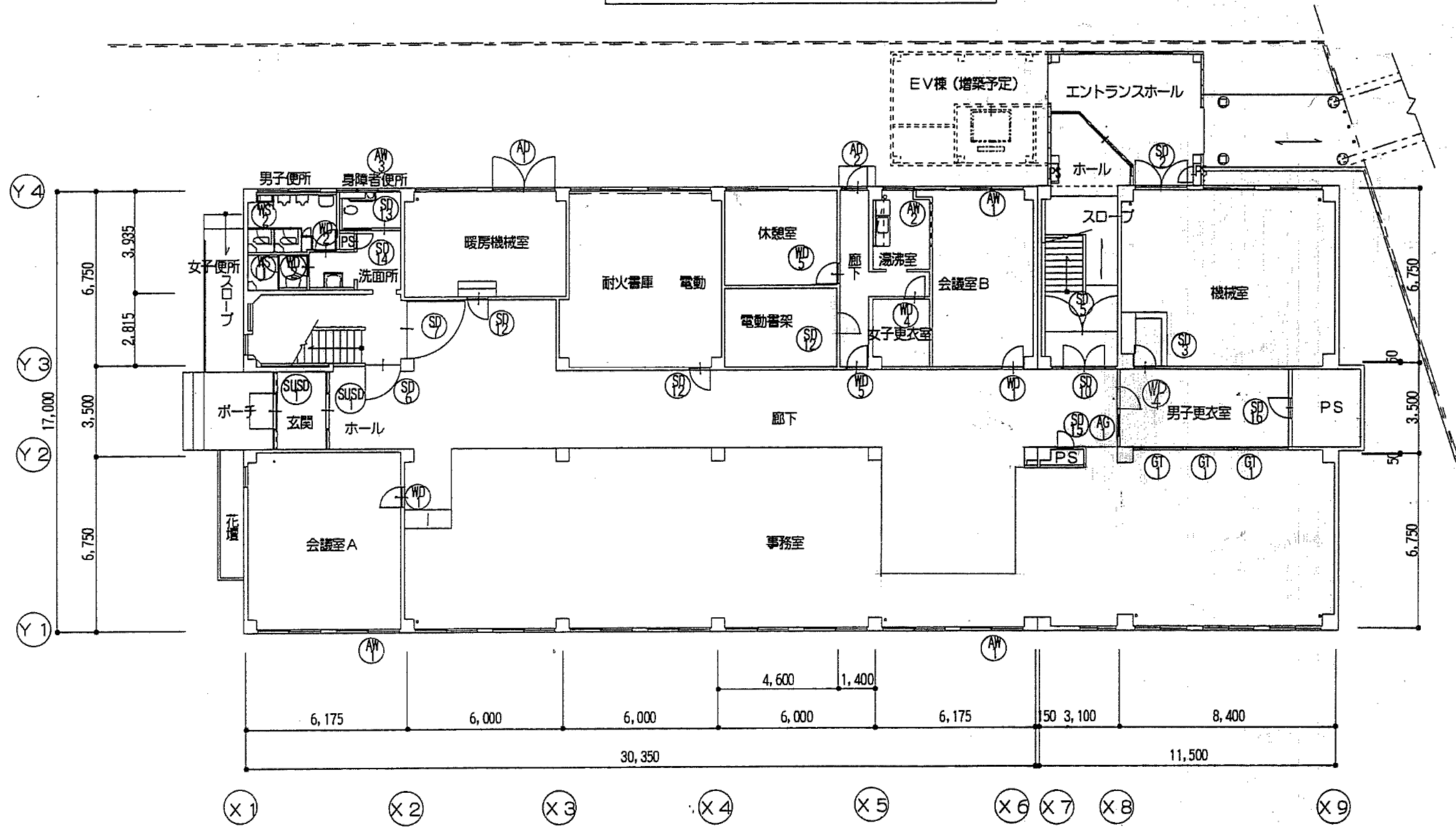
改修後 2階建具配置図 SC1:200
