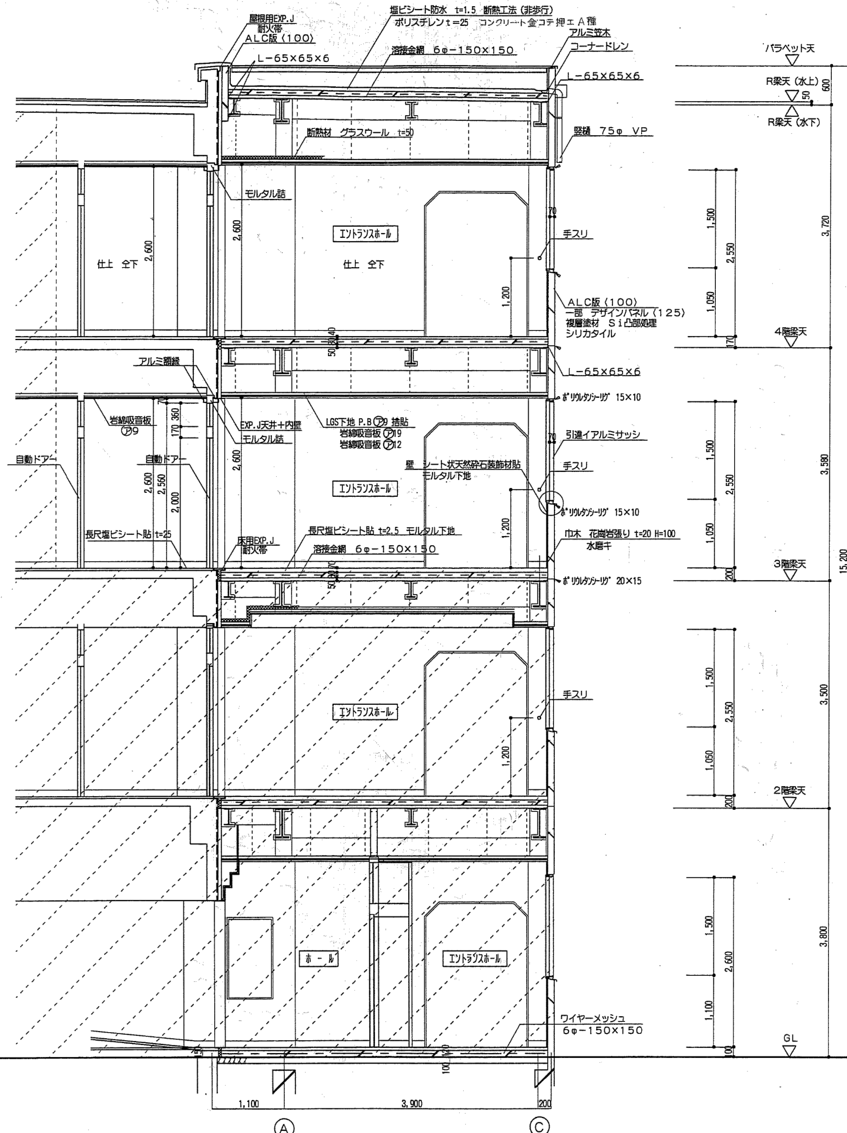
① ③ エントランスホール矩計図 SC1:50
