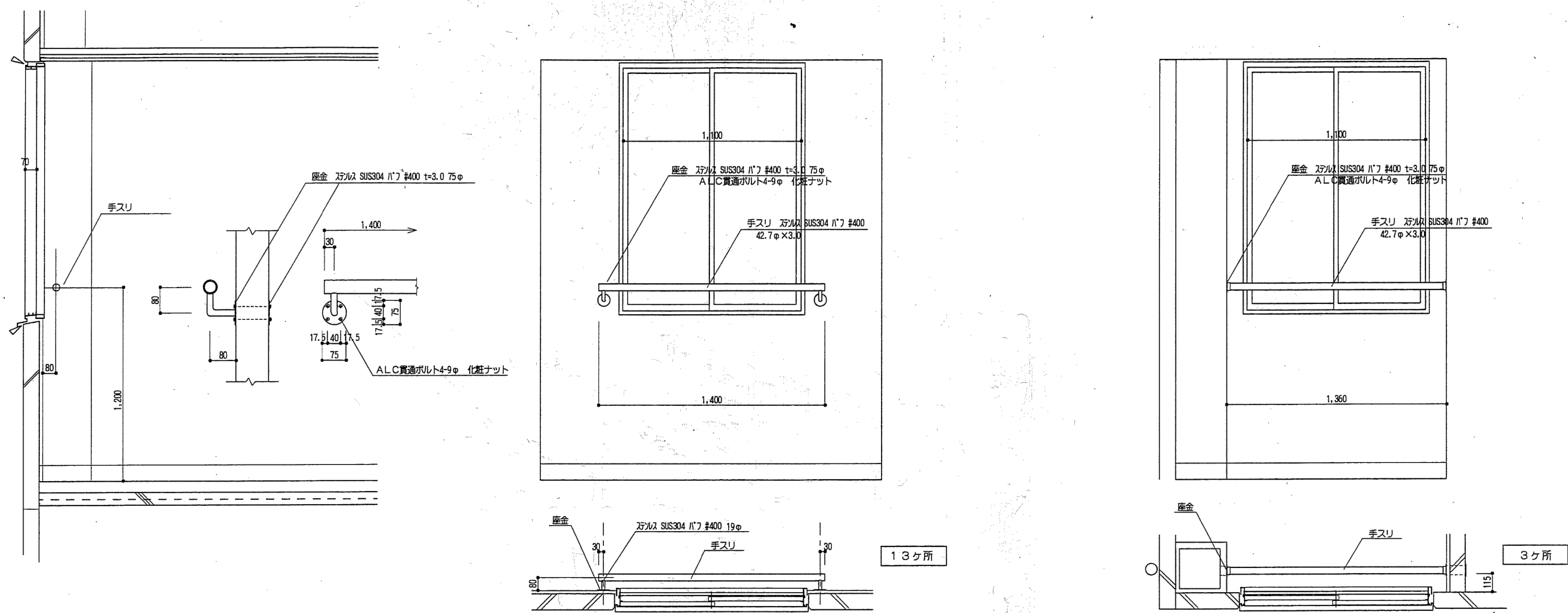
内部 手スリ詳細図 SC1:20
