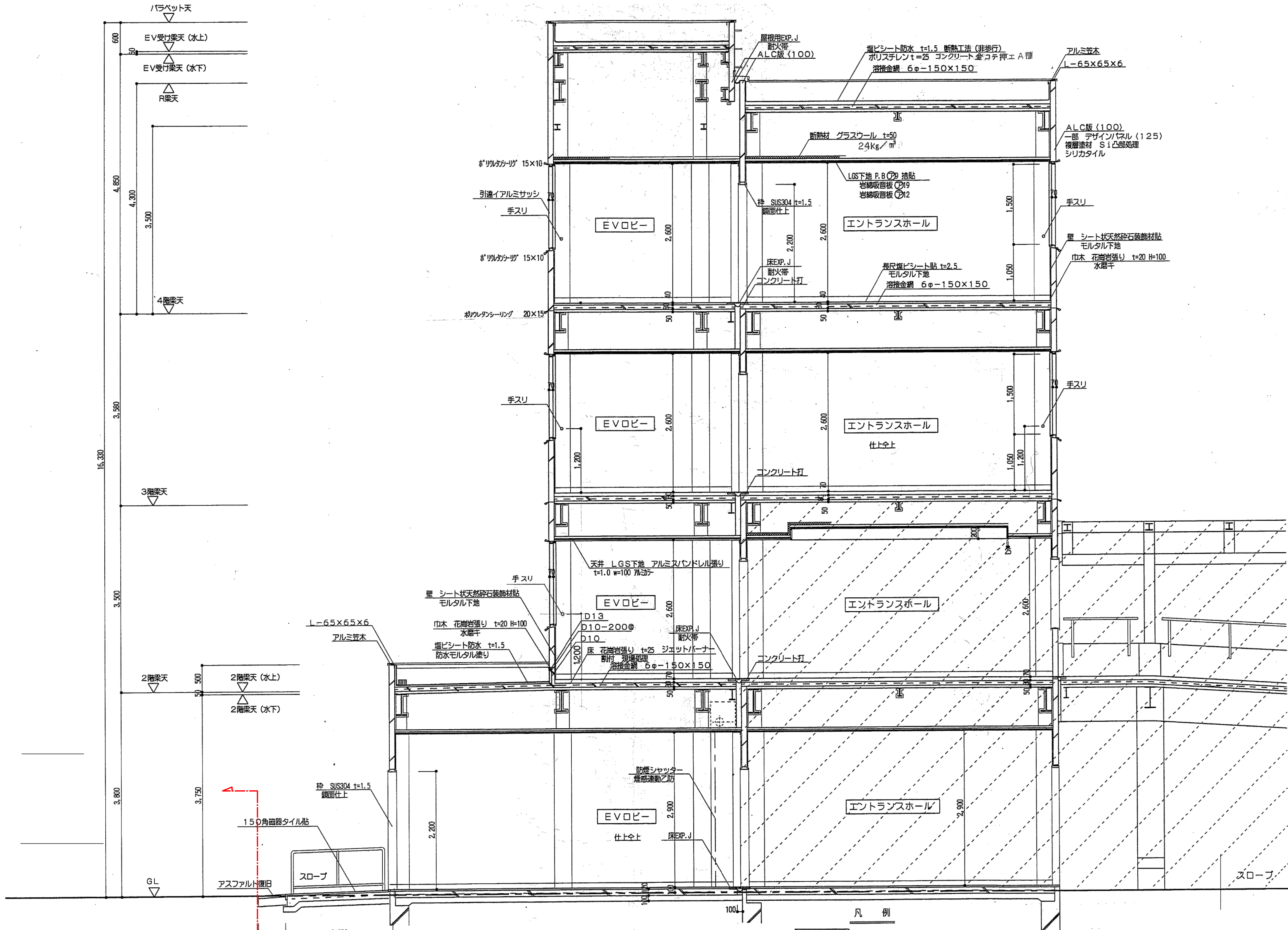
エントランスホール-EVOビー-矩計図 SC1:50
