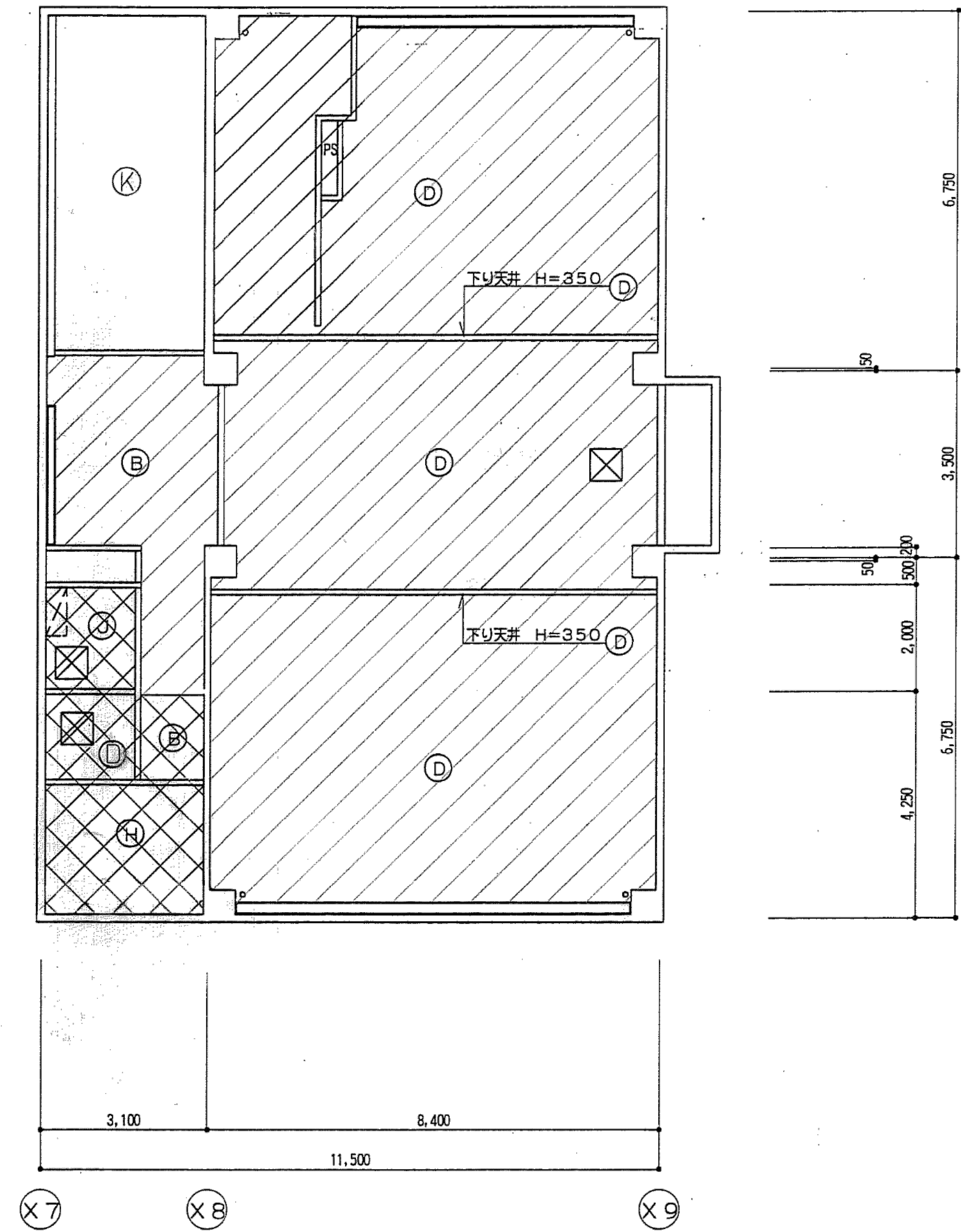
改修後 4階天井伏図 SC1:100
