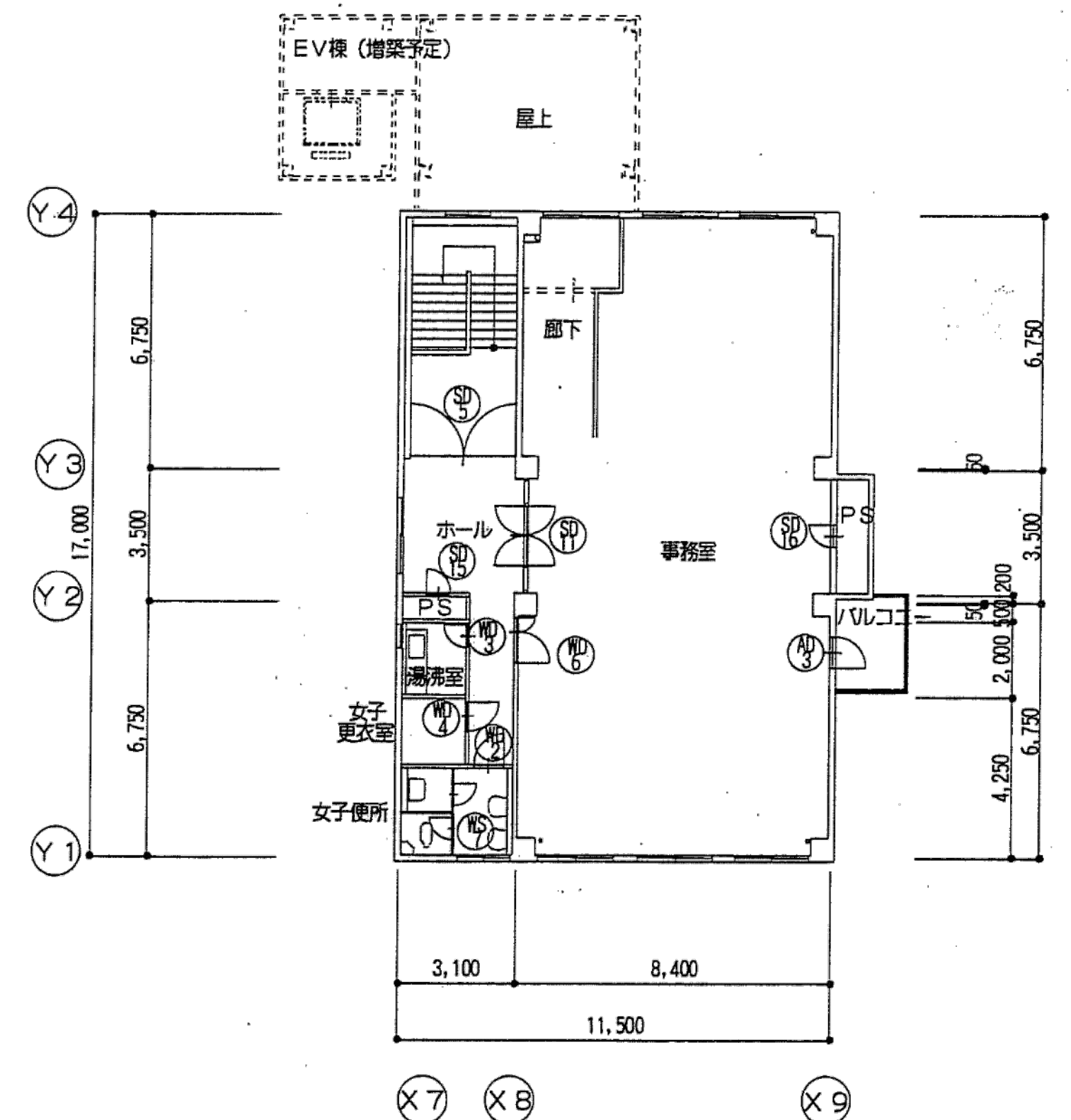
改修後 4階建具配置図 SC1:200
