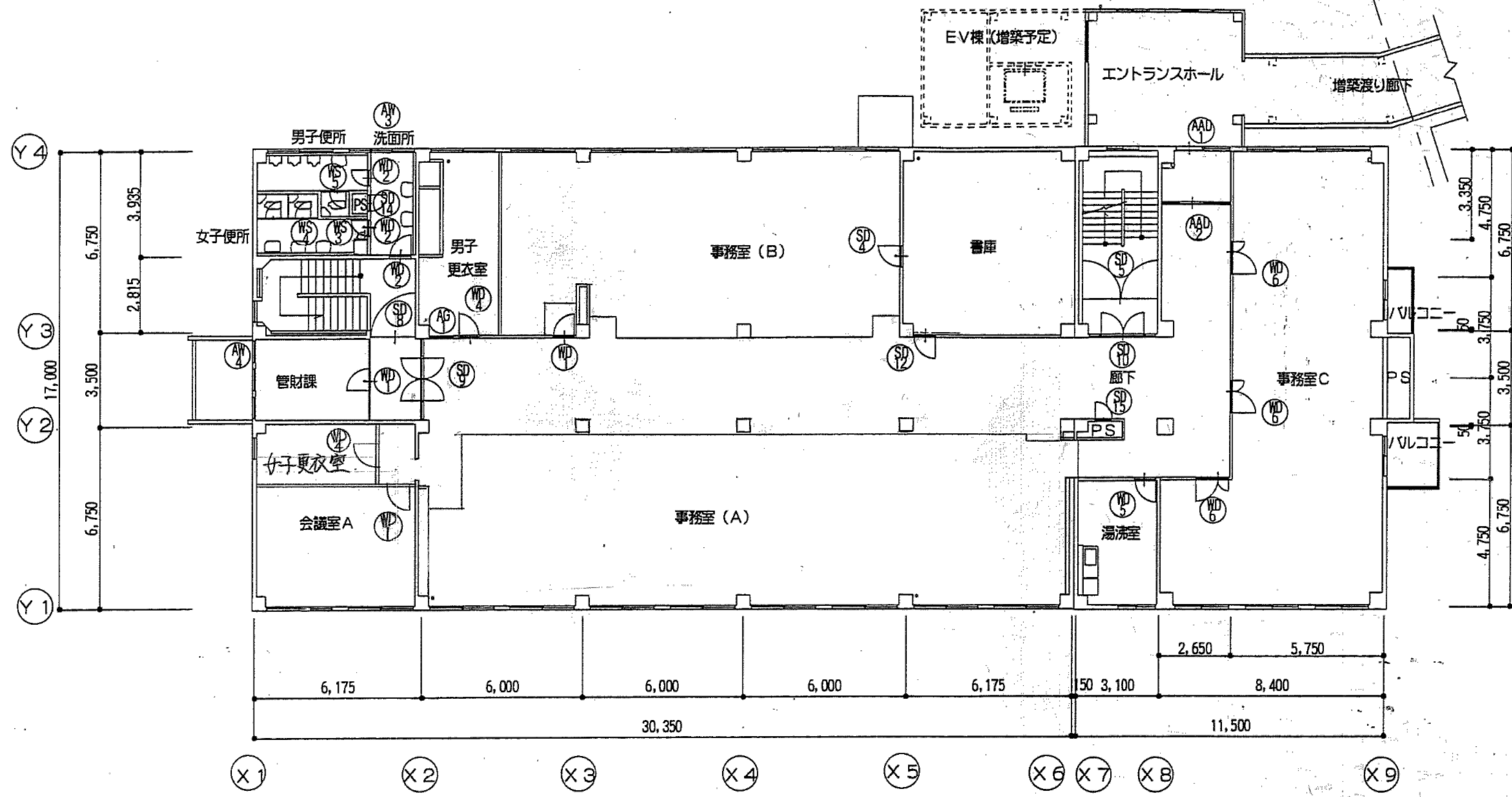
改修後 2階建具配置図 SC1:200
