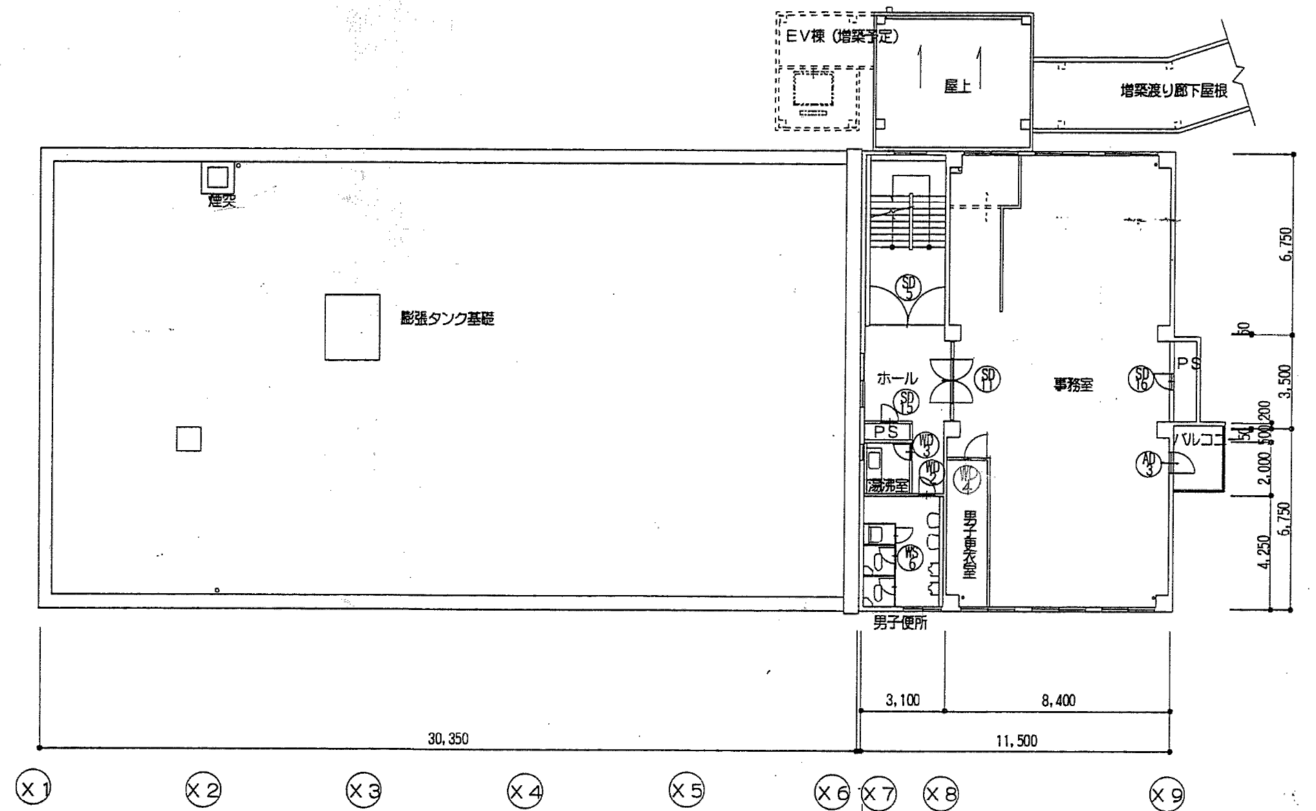
改修後 3階建具配置図 SC1:200
