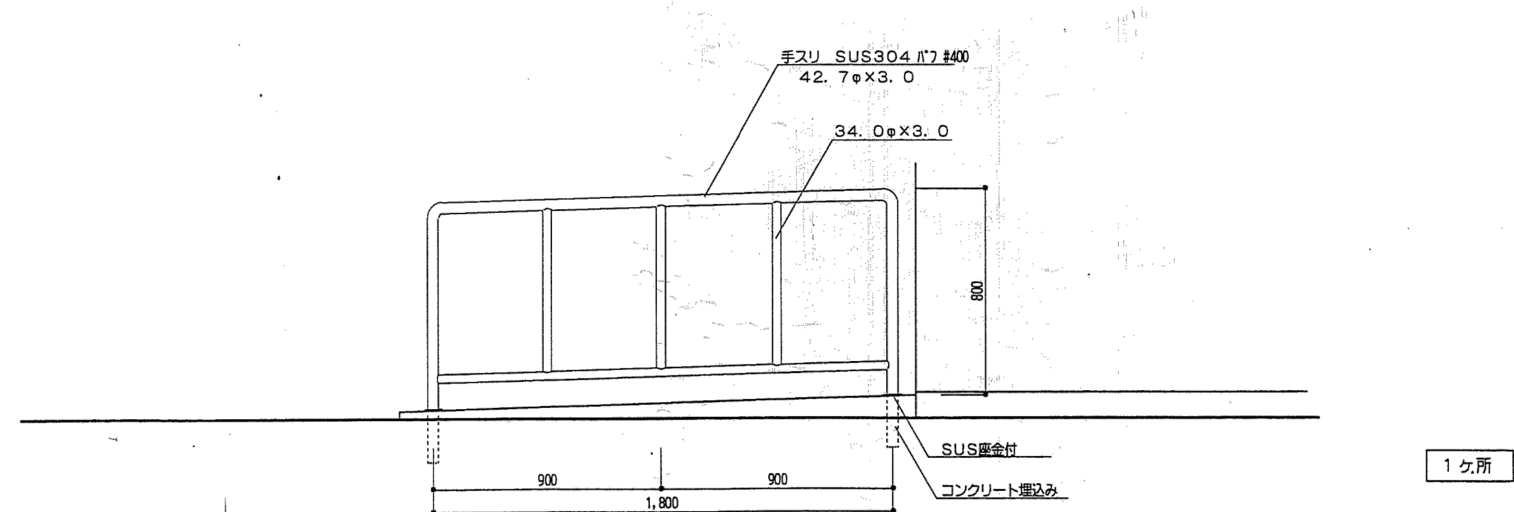
外部 手スリ詳細図 SC1:20
