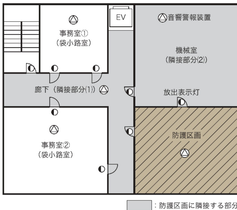
放出表示灯等の設置例（その1）
