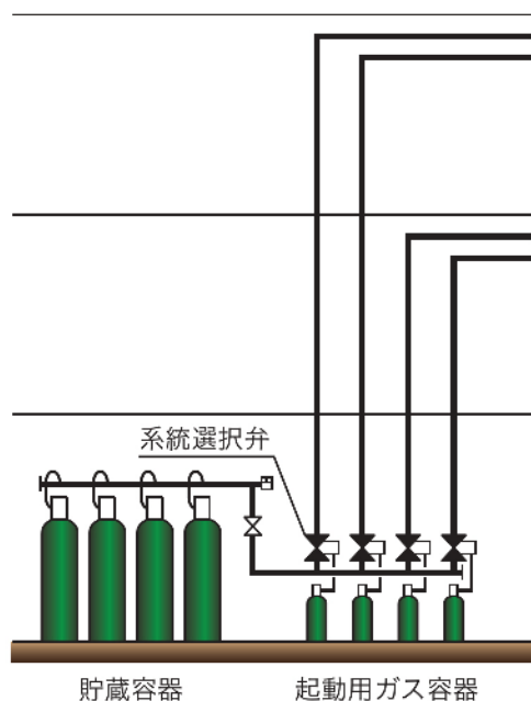
（一般的な配管方式の例）
