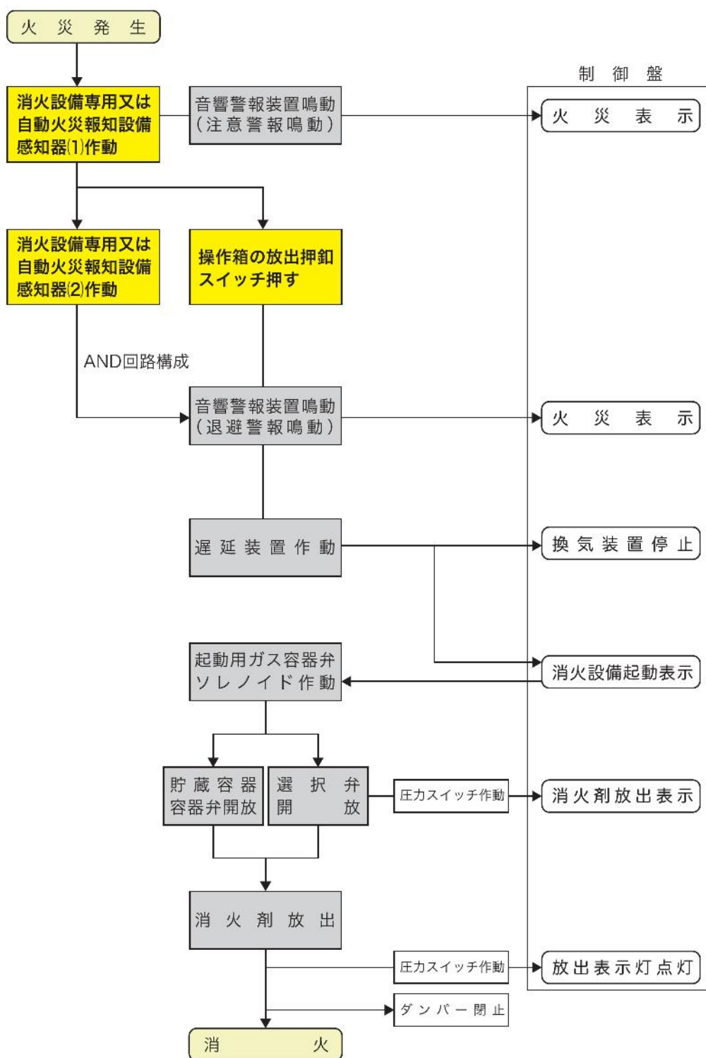
自動式の場合のフロー
