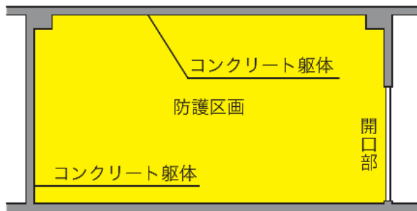
例1（壁及び床がコンクリート躯体である場合）
