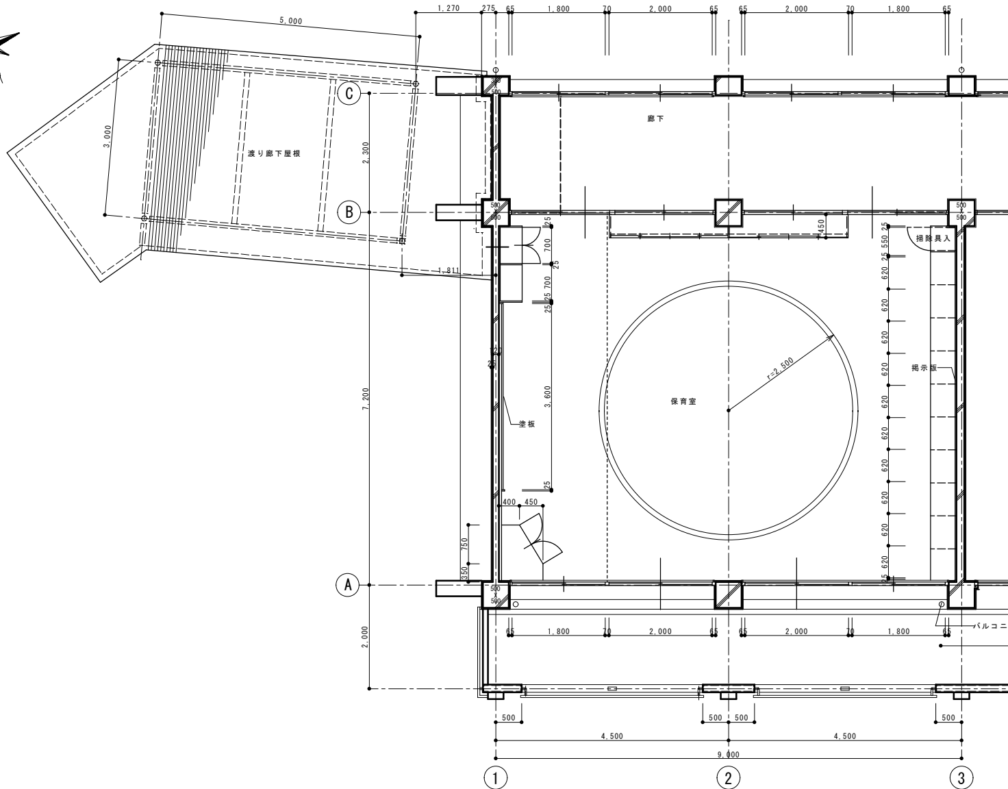
2階 平面詳細図
