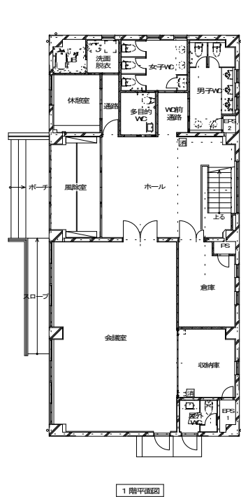
1 階平面図
