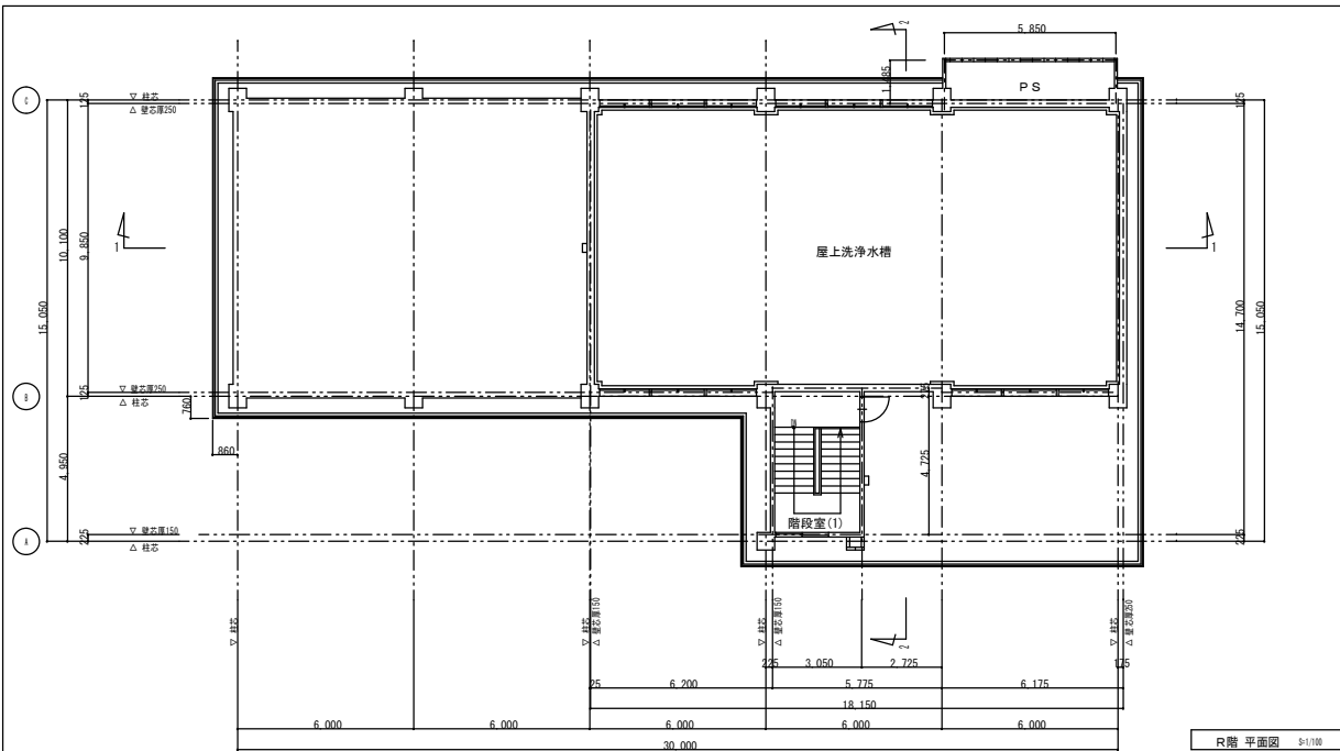
R階 平面図 ⑤-1/100
