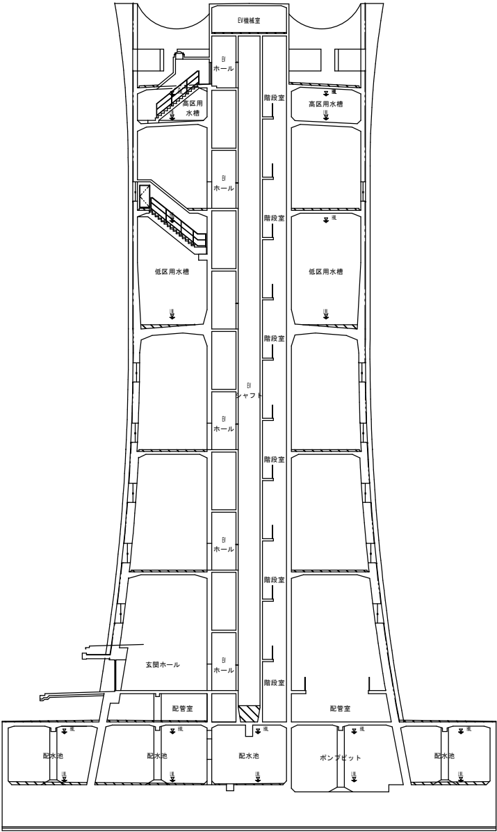
配水塔 1-1 断面図 S-1/100
