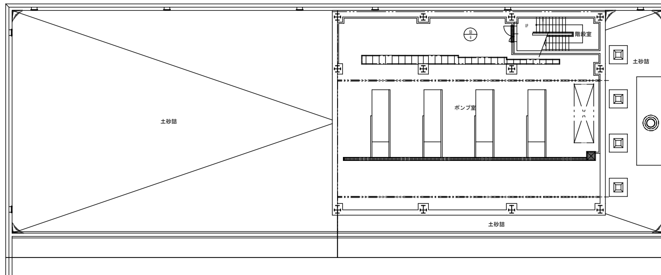
地階 建具配置図 3/1/100
