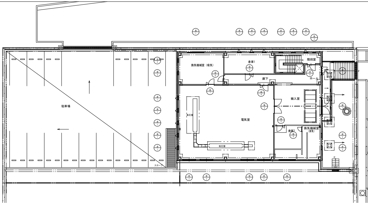
1階 建具配置図 3/1/100
