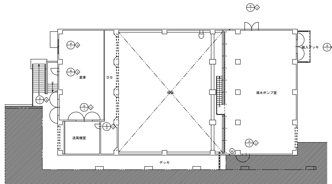
2階 建具配置図 ⑤-1/100
