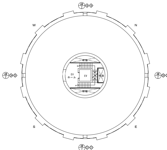
3階建具配置図 S=1/100
