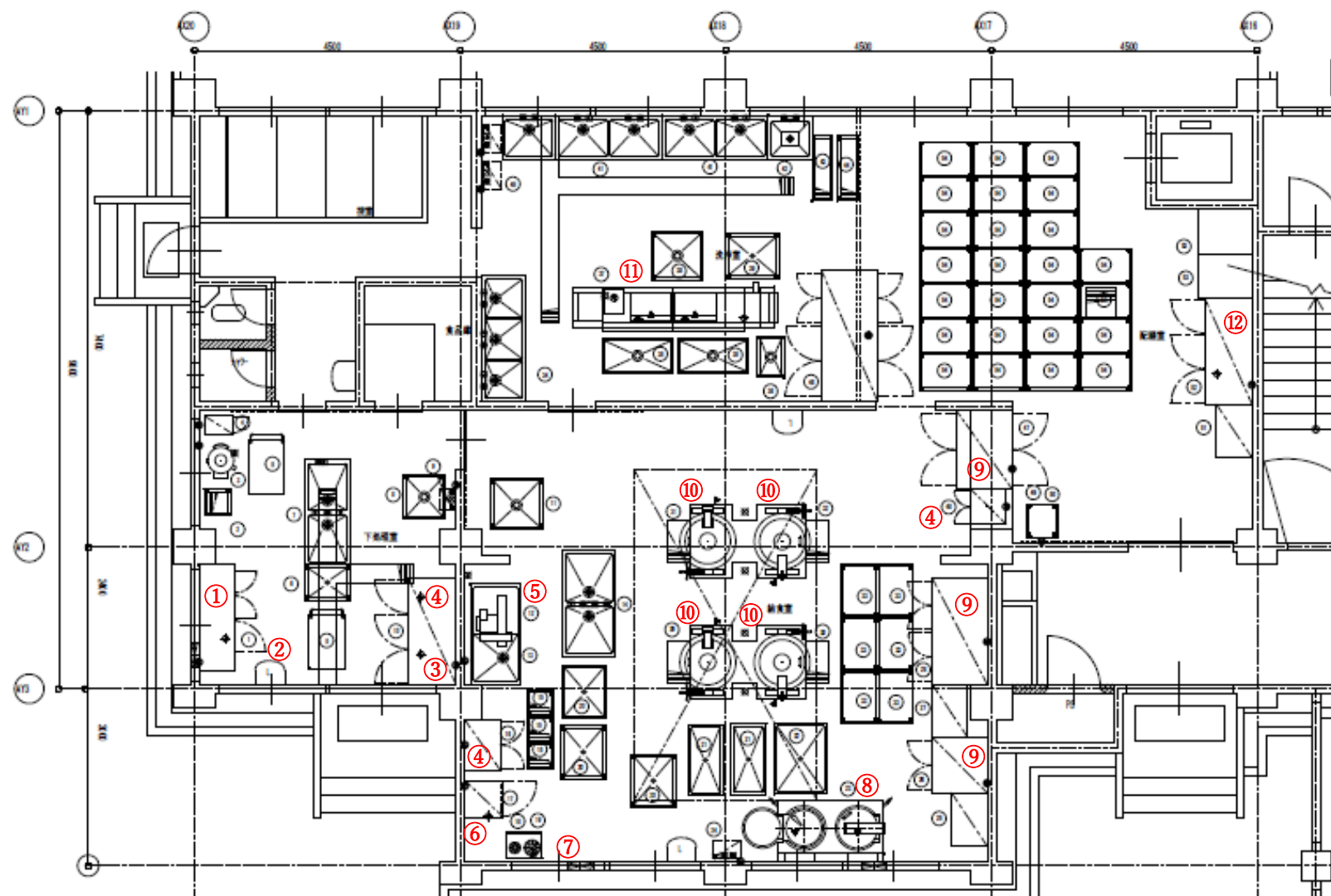
清水小学校設置機器配置図
