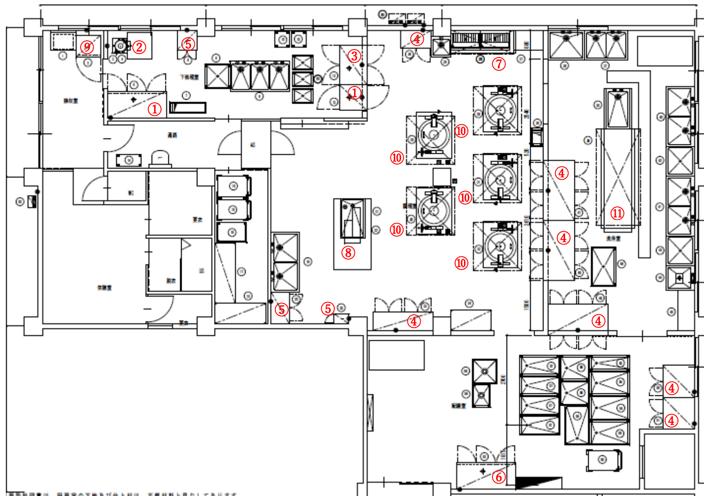
大久保小学校設置機器配置図
