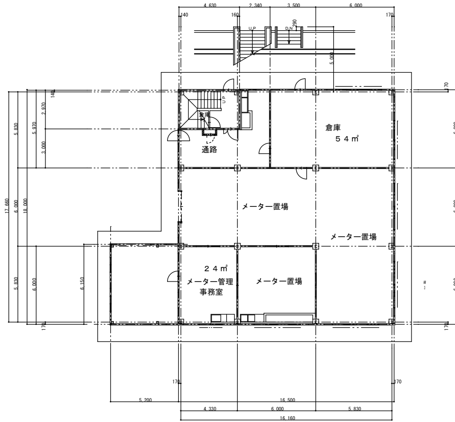
サービスセンター棟 1 階平面図
