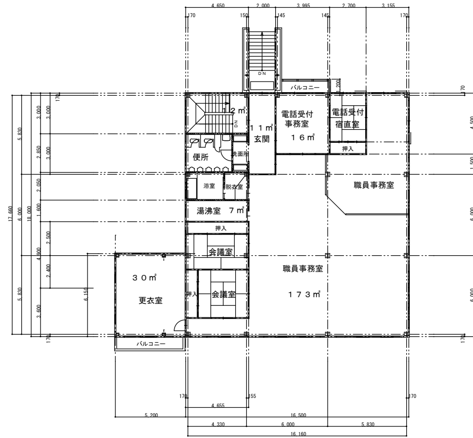
サービスセンター棟 2 階平面図
