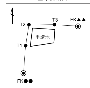
基準点網図
