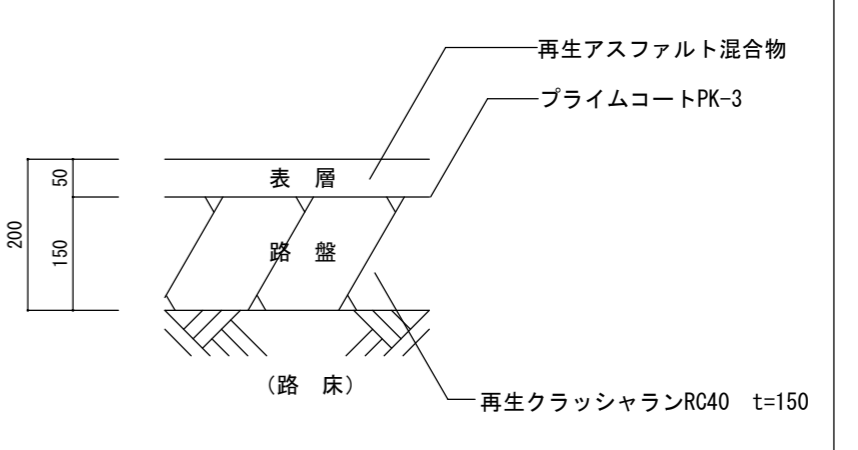
② インターロッキングブロック舗装 1/10
