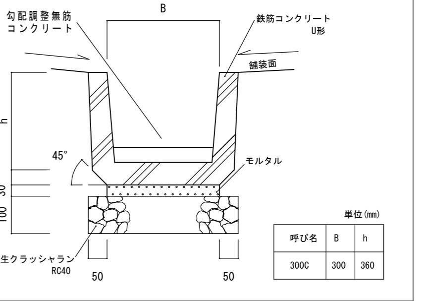
② U字溝 1/10
