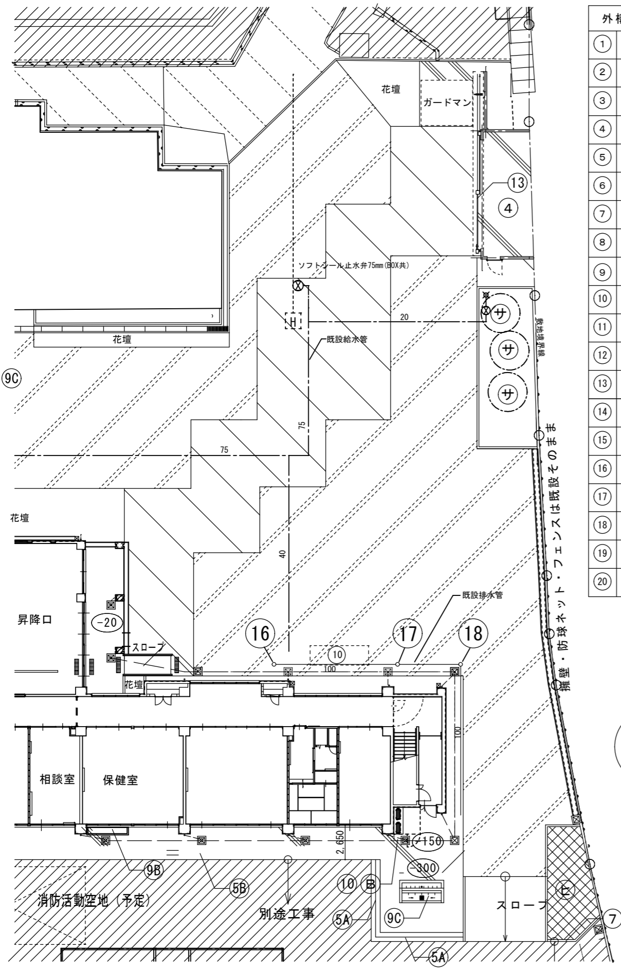
既設外構図 S=1/300
