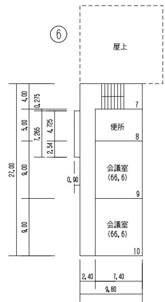
3階平面図
