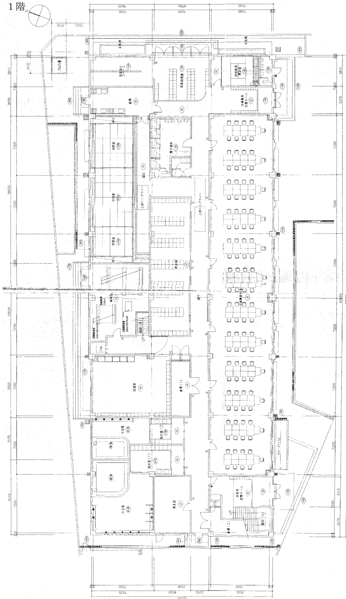
1階平面図
