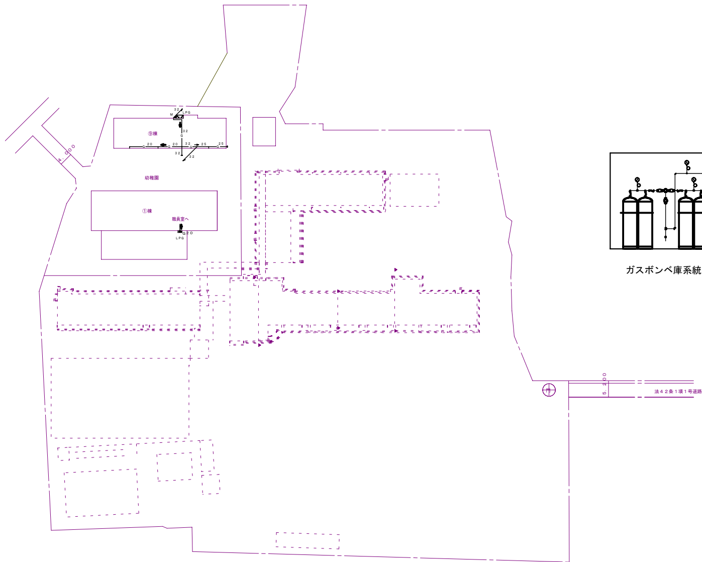
配置図 (ガス) 1/600
