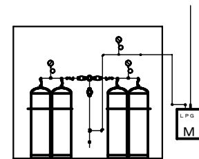
ガスボンベ庫系統図
