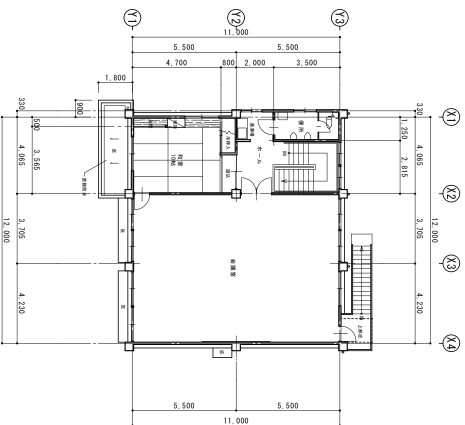
2階平面図
