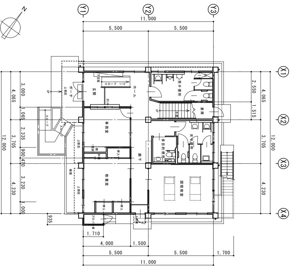
1階平面図
