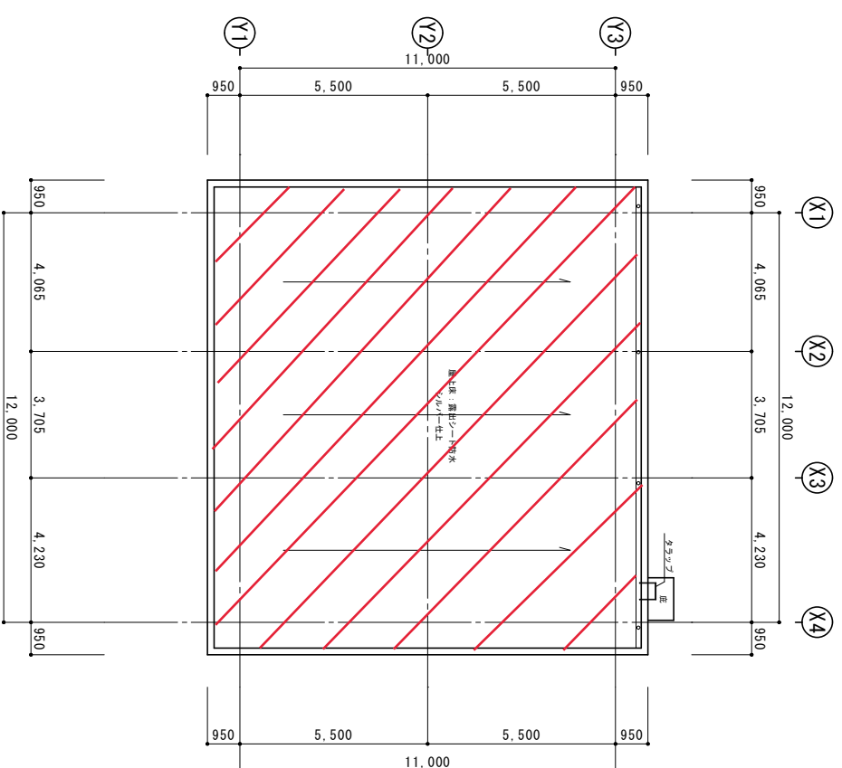
屋根伏図
