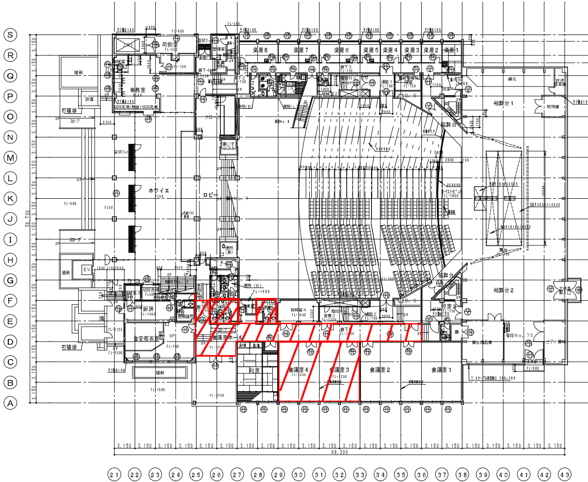
1階平面図 1/200
